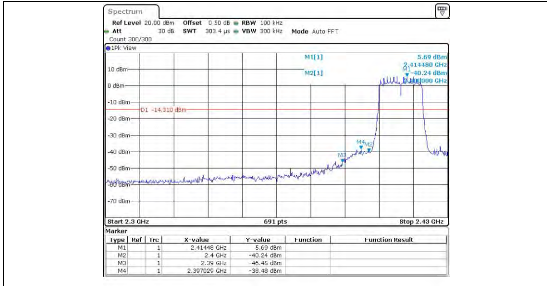
11G_Ant0_Low_2412
