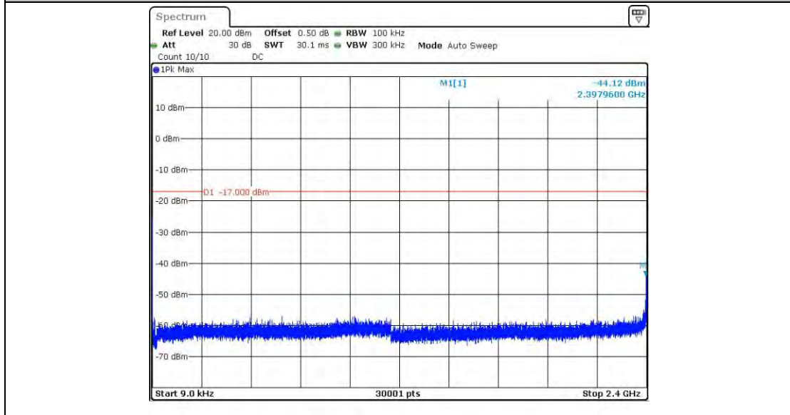
11B_Ant0_2412_0.009~2400
