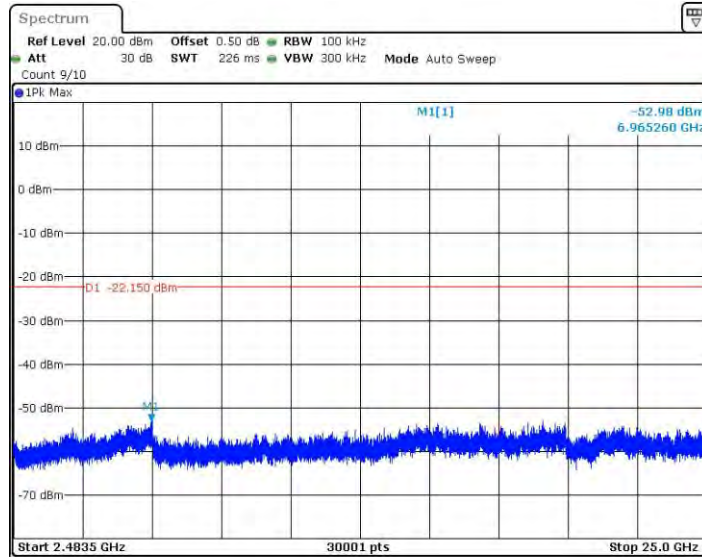
11AX40SISO_Ant0_2422_2483.5~25000
