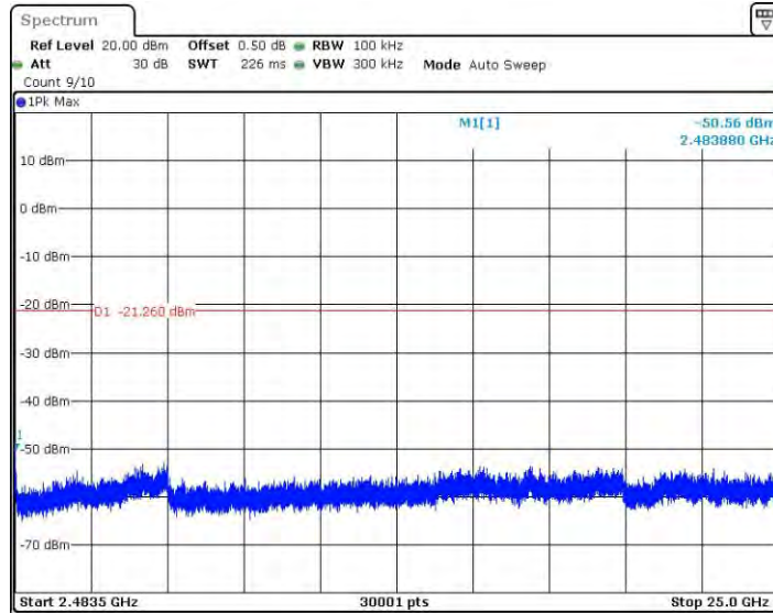
11AX40SISO_Ant1_2437_2483.5~25000
