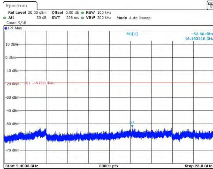
11AX20SISO_Ant0_2437_2483.5~25000
