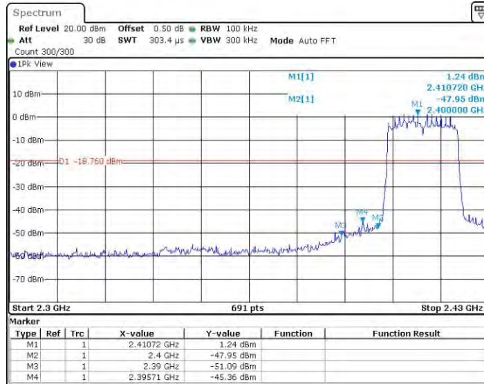
11AX20SISO_Ant0_Low_2412
