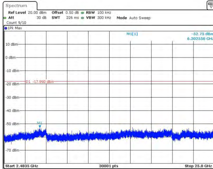
11AX20SISO_Ant1_2437_2483.5~25000
