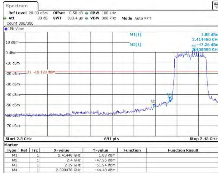
11AX20SISO_Ant1_Low_2412
