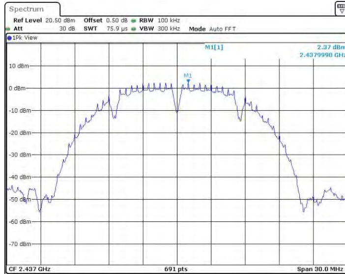
11B_Ant0_2437_0~Reference
