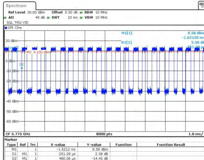
11AC80MIMO_Ant1_5775
