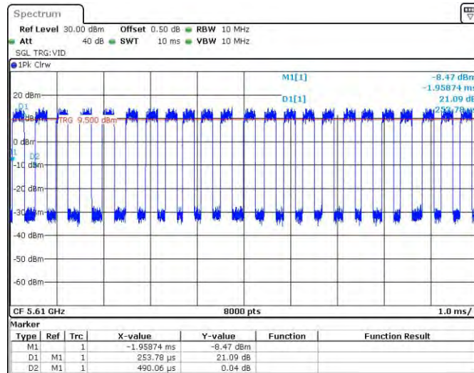
11AC80MIMO_Ant2_5610
