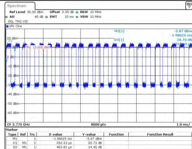
11AC80MIMO_Ant2_5775
