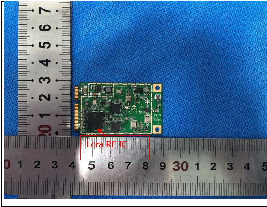
EUT-5
