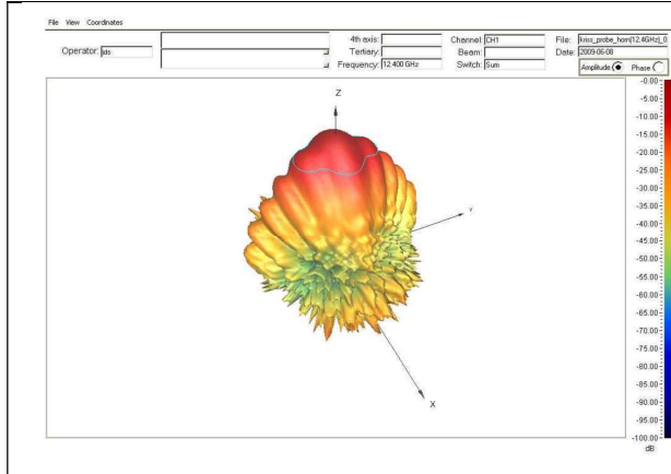
▲ 측정결과 (3D Amplitude)
