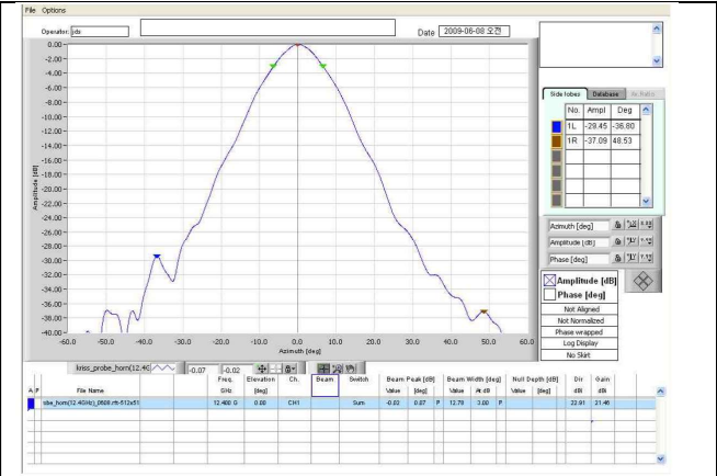
▲ 측정결과 (Cartesian Azimuth)
