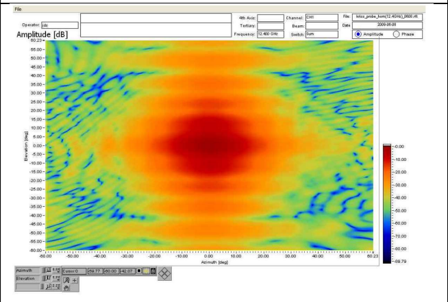
▲ 측정결과 (Intensity Amplitude)
