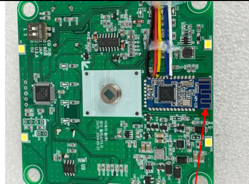
Antenna
