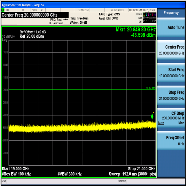
BLE_1M-Ant1-2480-19000~21000-PASS
