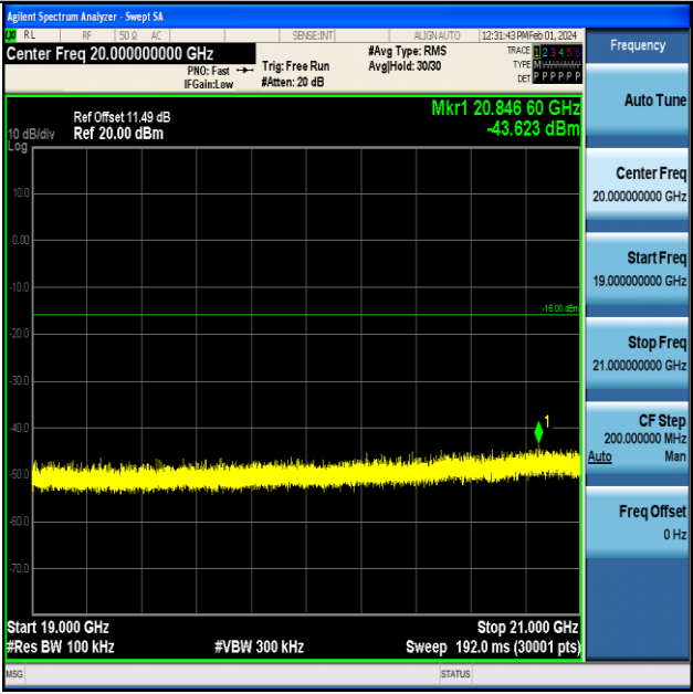
DH5-Ant1-2480-19000~21000-PASS
