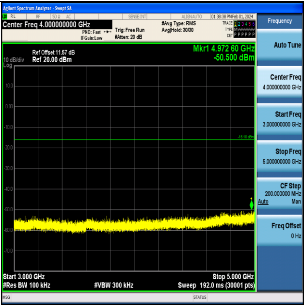
3DH5-Ant1-2441-3000~5000-PASS
