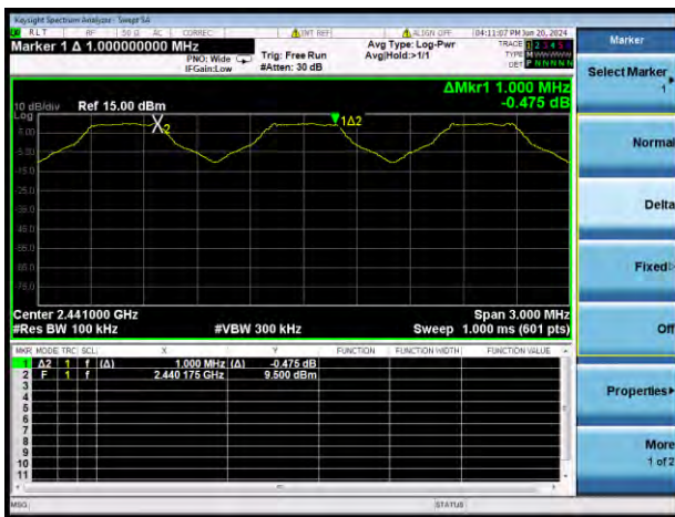
GFSK
