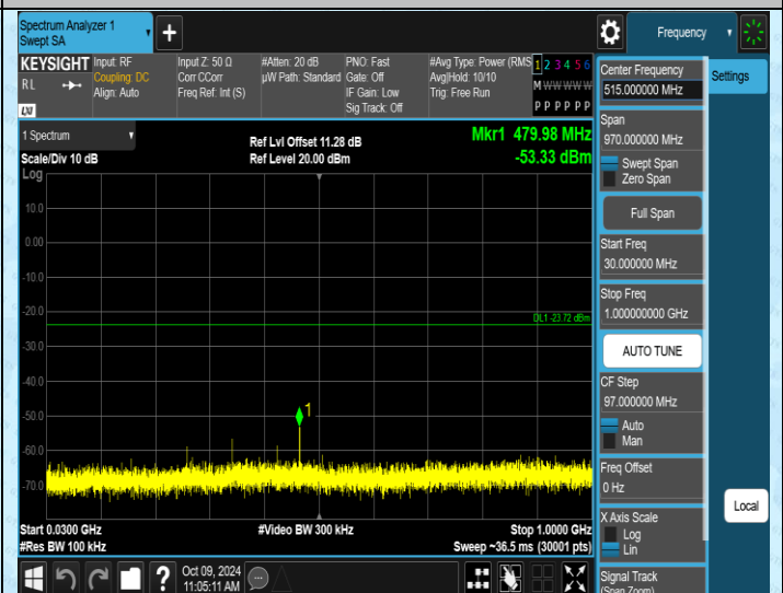
11G-Ant1-2412-30~1000-PASS
