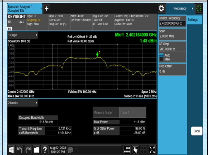
TX-Ant2-2402
