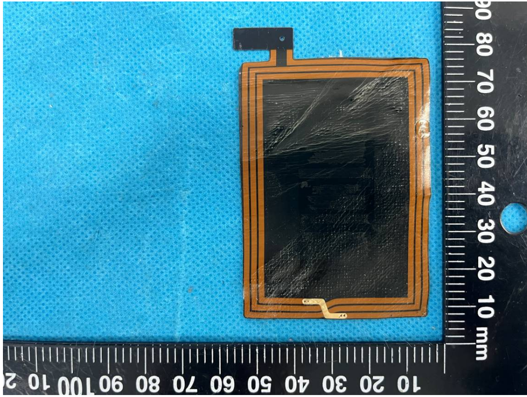
NFC Antenna
