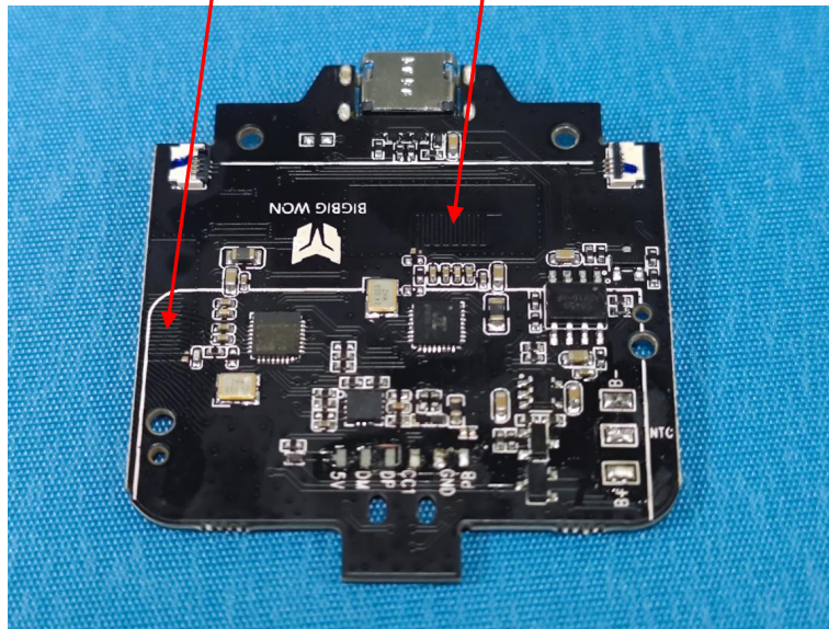
PCB Antenna (2.4G)
