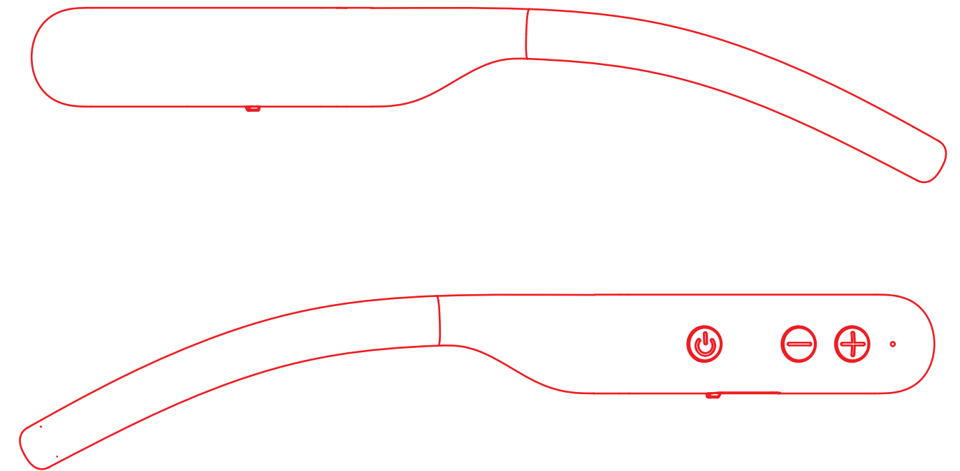
B113 耳机壳料外侧面丝印位置区域
