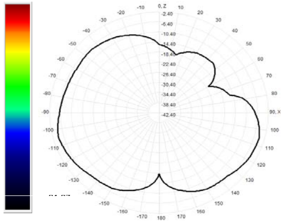
907.0MHz Total(E1-XZ), Max=-4.37dBi
