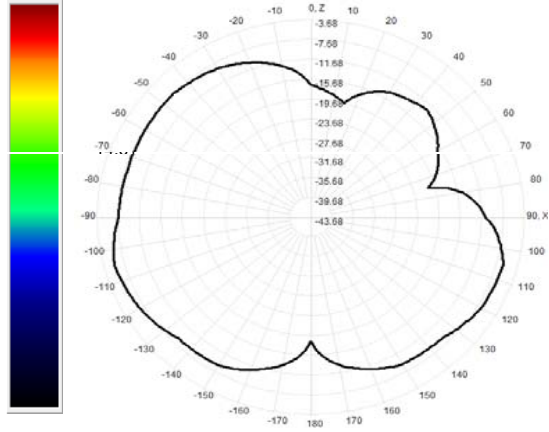
927.0MHz Total(E1-XZ), Max= -5.72dBi
