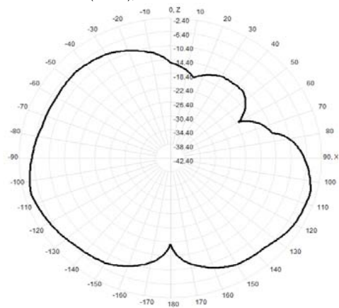
902.0MHz Total(E1-XZ), Max=-4.24dBi
