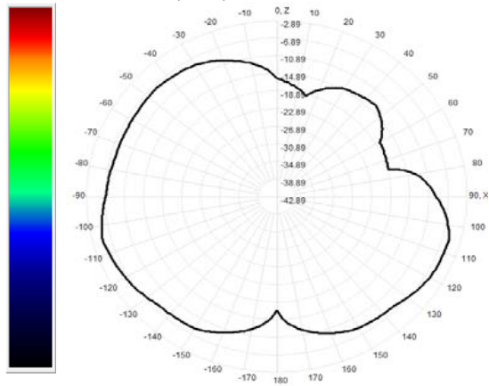
917.0MHz Total(E1-XZ), Max= -5.08dBi
