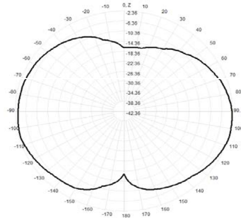
906.0MHz Total(E2-YZ), Max=-2.36dBi
