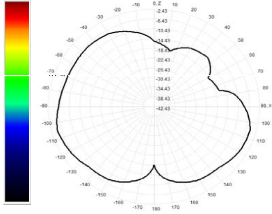
912.0MHz Total(E1-XZ), Max= -4.74dBi
