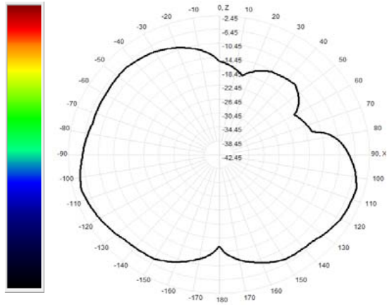
911.0MHz Total(E1-XZ), Max= -4.62dBi
