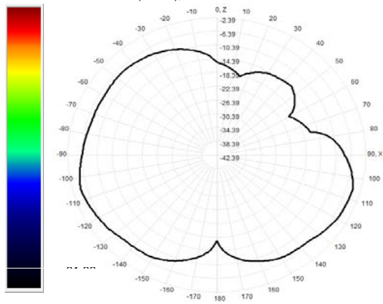
910.0MHz Total(E1-XZ), Max=-4.60dBi
