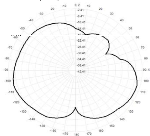
903.0MHz Total(E1-XZ), Max=-4.34dBi
