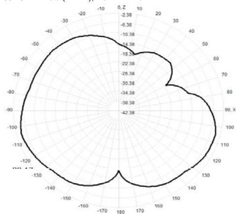
904.0MHz Total(E1-XZ), Max=-4.27dBi
