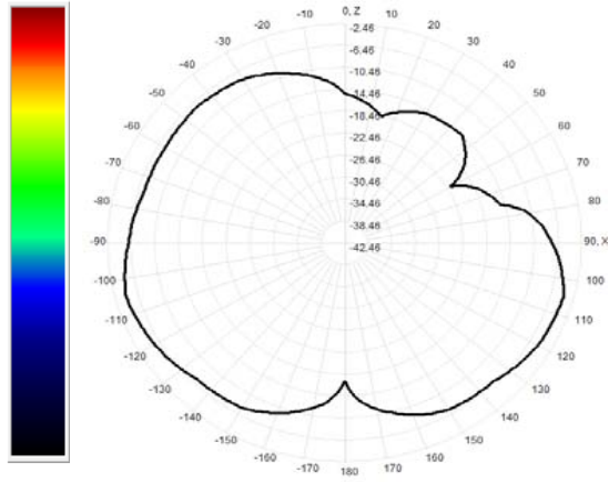
905.0MHz Total(E1-XZ), Max=-4.35dBi
