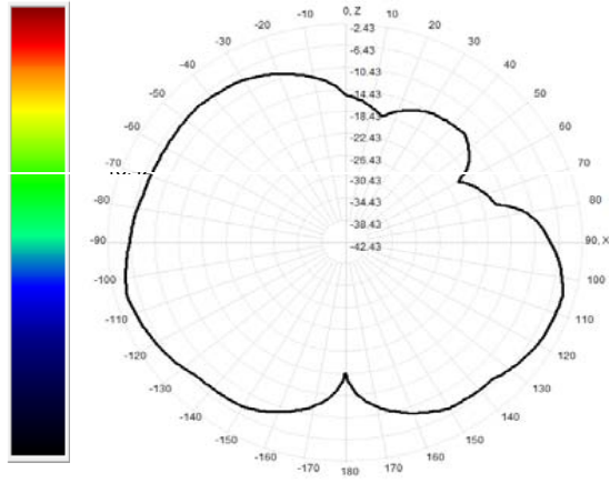
909.0MHz Total(E1-XZ), Max=-4.45dBi
