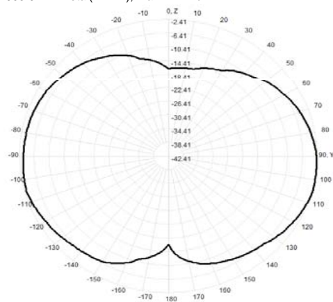
903.0MHz Total(E2-YZ), Max=-2.41dBi
