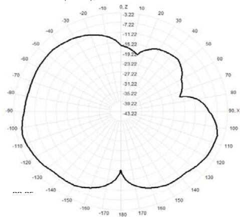
922.0MHz Total(E1-XZ), Max= -5.36dBi
