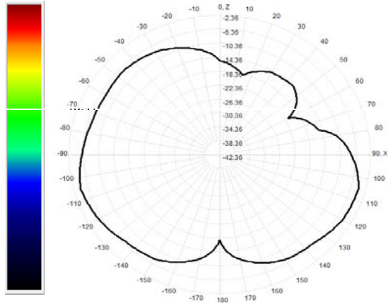
906.0MHz Total(E1-XZ), Max=-4.32dBi
