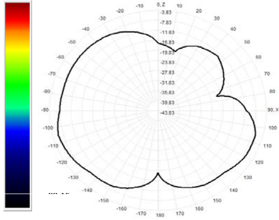
928.0MHz Total(E1-XZ), Max= -5.95dBi
