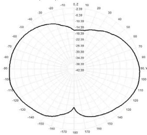
910.0MHz Total(E2-YZ), Max=-2.39dBi
