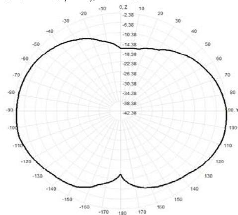
904.0MHz Total(E2-YZ), Max=-2.38dBi
