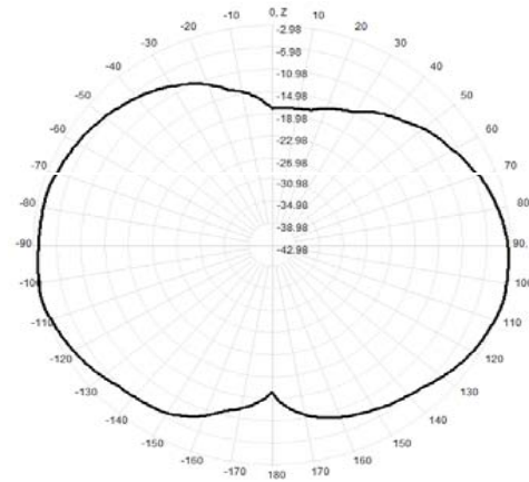
918.0MHz Total(E2-YZ), Max= -2.98dBi
