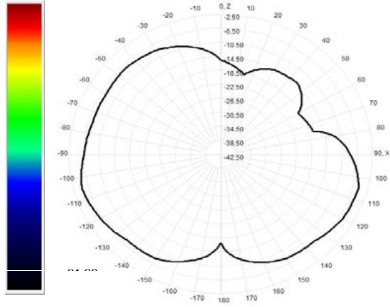
913.0MHz Total(E1-XZ), Max= -4.75dBi
