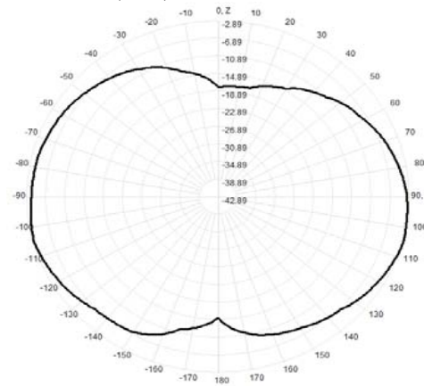
917.0MHz Total(E2-YZ), Max= -2.89dBi
