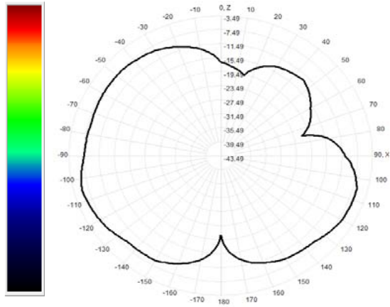
926.0MHz Total(E1-XZ), Max= -5.72dBi
