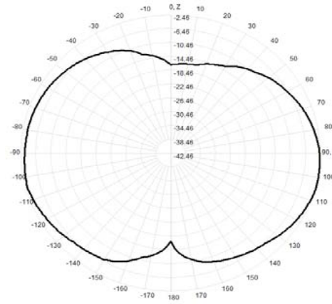
905.0MHz Total(E2-YZ), Max=-2.46dBi
