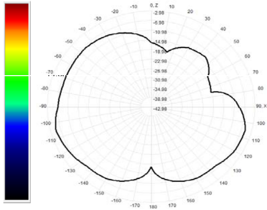
918.0MHz Total(E1-XZ), Max= -5.14dBi
