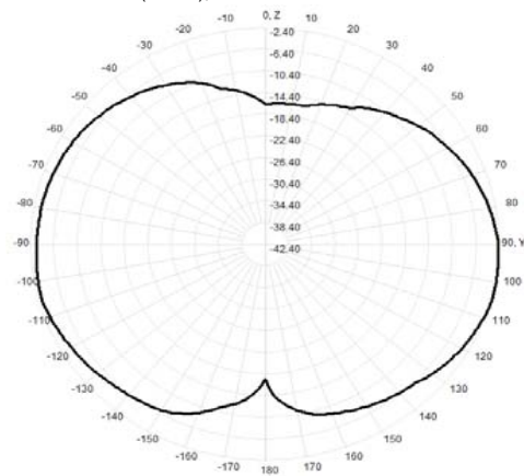
902.0MHz Total(E2-YZ), Max=-2.40dBi
