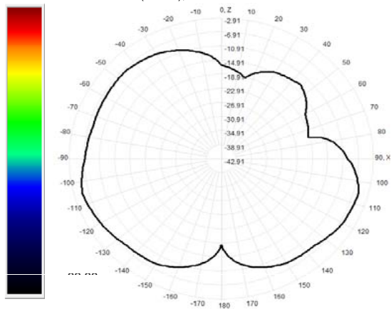
919.0MHz Total(E1-XZ), Max= -5.16dBi
