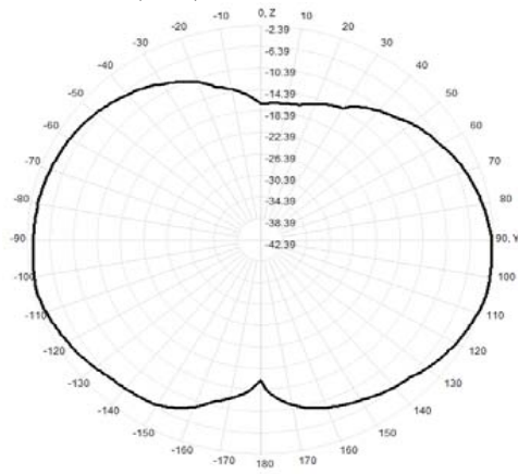
908.0MHz Total(E2-YZ), Max=-2.39dBi
