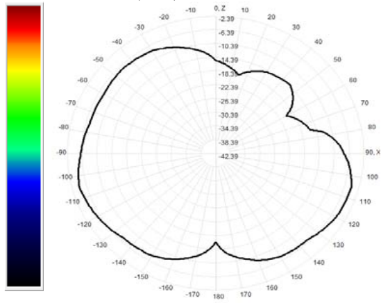
908.0MHz Total(E1-XZ), Max=-4.41dBi
