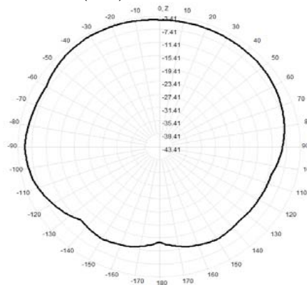
904.0MHz Total(E2-YZ), Max= -4.17dBi
