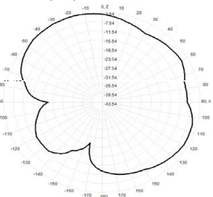
903.0MHz Total(E1-XZ), Max= -3.54dBi
