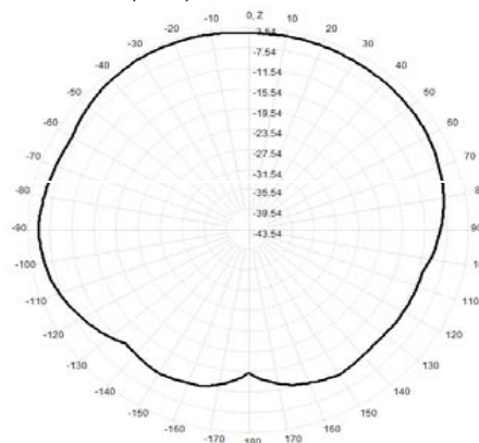
903.0MHz Total(E2-YZ), Max= -4.21dBi
