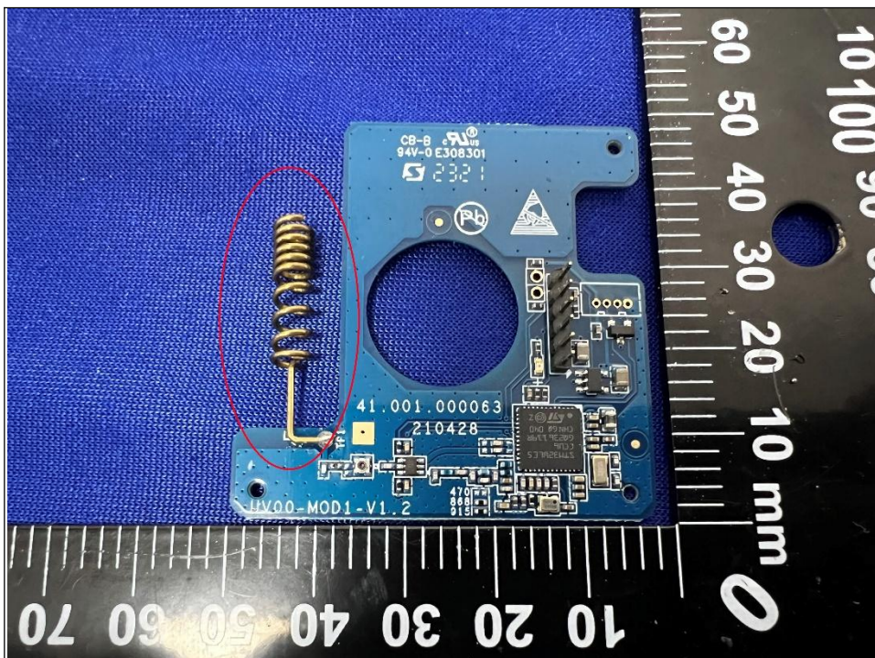
LORA ANTENNA
