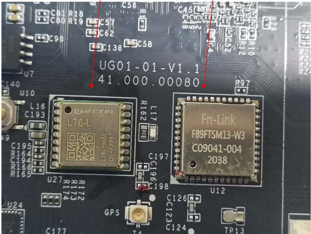
GPS Module
