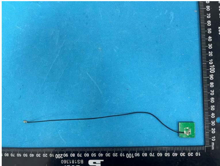
WWAN Module
