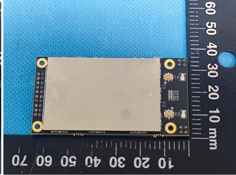
Lora Module
