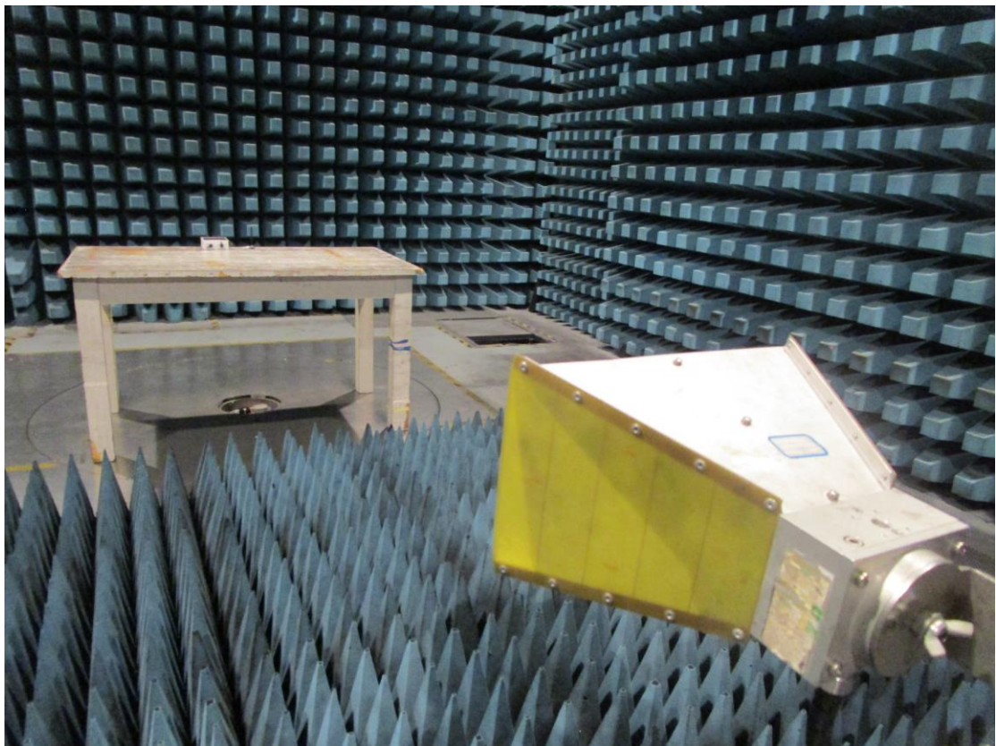
RE_Above 1GHz_External Ant
