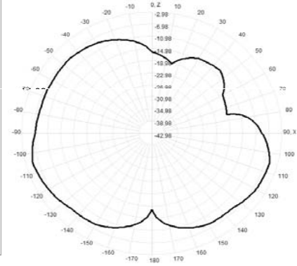
919.0MHz Total(E1-XZ), Max= -5.16dBi
