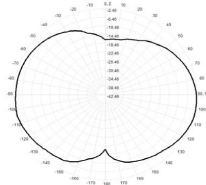
905.0MHz Total(E2-YZ), Max= -2.46dBi
