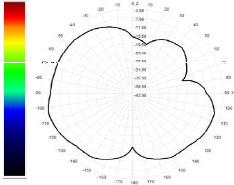
928.0MHz Total(E1-XZ), Max= -5.95dBi
