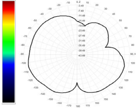
926.0MHz Total(E1-XZ), Max= -5.72dBi
