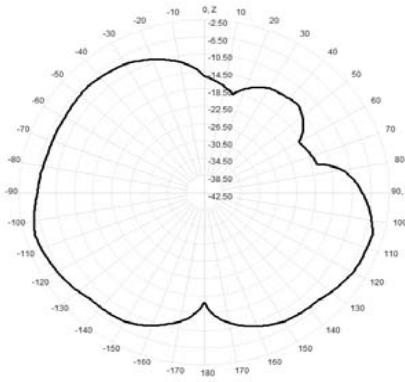
913.0MHz Total(E1-XZ), Max= -4.75dBi
