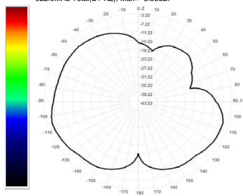
922.0MHz Total(E1-XZ), Max= -5.36dBi
