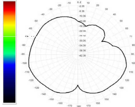
906.0MHz Total(E1-XZ), Max= -4.32dBi
