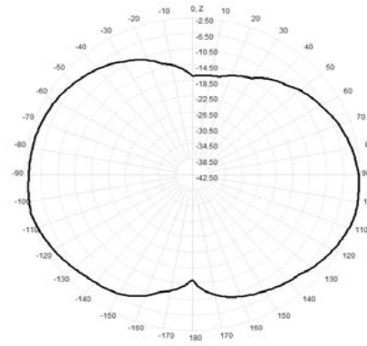
913.0MHz Total(E2-YZ), Max= -2.50dBi
