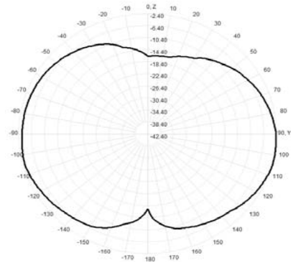
902.0MHz Total(E2-YZ), Max=-2.40dBi
