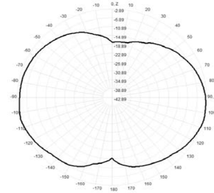
917.0MHz Total(E2-YZ), Max= -2.89dBi
