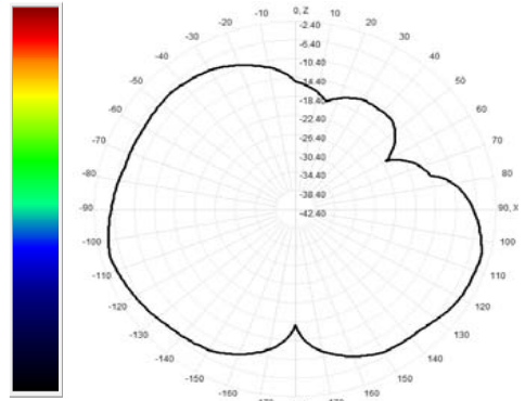
902.0MHz Total(E1-XZ), Max=-4.24dBi
