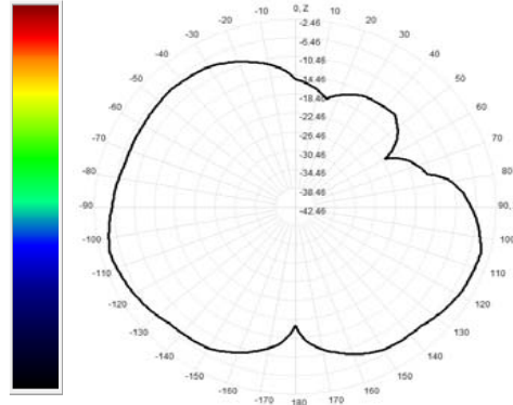
905.0MHz Total(E1-XZ), Max= -4.35dBi
