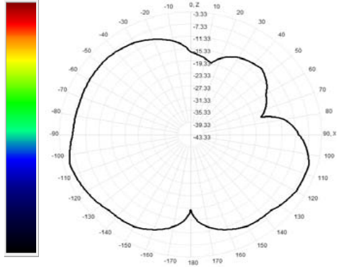
923.0MHz Total(E1-XZ), Max= -5.34dBi
