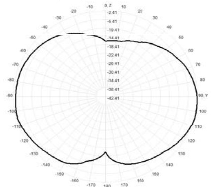
903.0MHz Total(E2-YZ), Max=-2.41dBi
