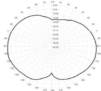
906.0MHz Total(E2-YZ), Max= -2.36dBi
