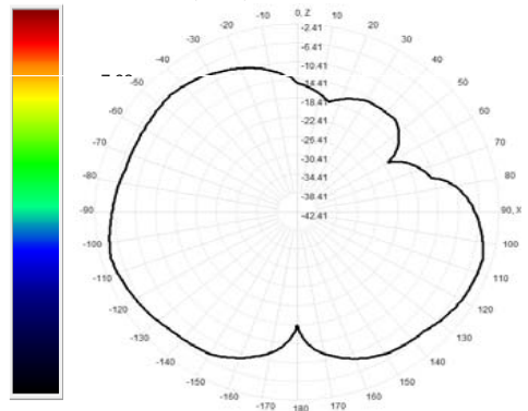
903.0MHz Total(E1-XZ), Max=-4.34dBi
