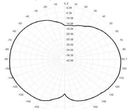
904.0MHz Total(E2-YZ), Max=-2.38dBi
