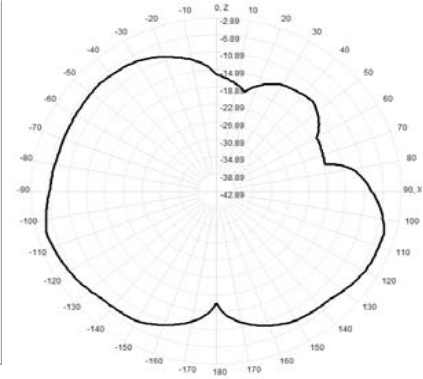
917.0MHz Total(E1-XZ), Max= -5.08dBi
