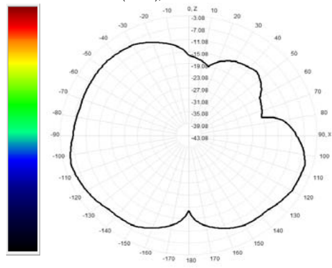
921.0MHz Total(E1-XZ), Max= -5.30dBi
