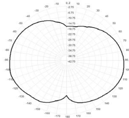
916.0MHz Total(E2-YZ), Max= -2.75dBi
