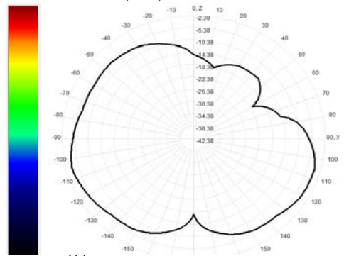
904.0MHz Total(E1-XZ), Max=-4.27dBi
