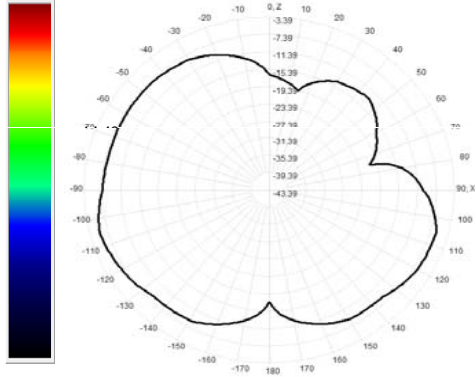
925.0MHz Total(E1-XZ), Max= -5.57dBi
