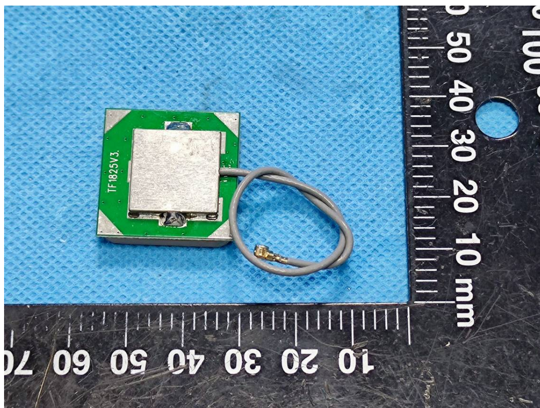
GPS Antenna
