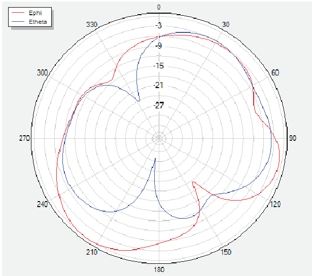
Theta=90 freq=2400MHz
