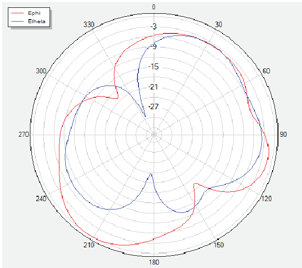
Theta=90 freq=2500MHz
