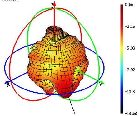
930MHz 3D_Graphs
