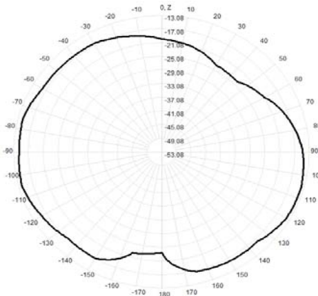
914.0MHz Total(E2-YZ), Max= -14.06dBi
