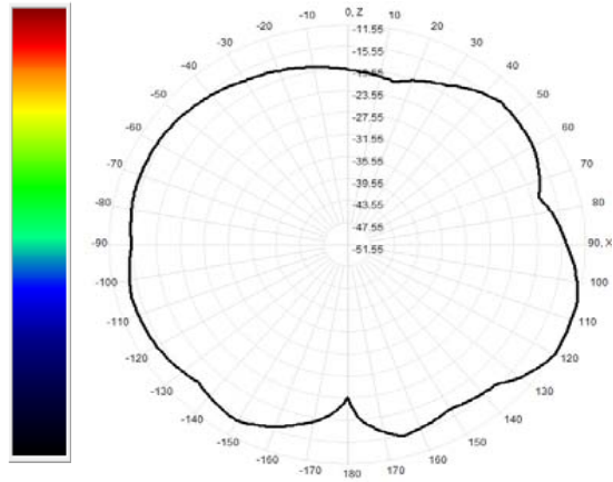
923.0MHz Total(E1-XZ), Max= -11.55dBi
