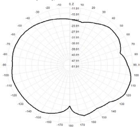
920.0MHz Total(E1-XZ), Max= -11.91dBi
