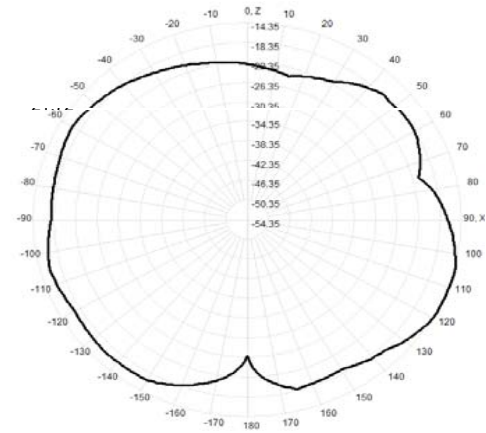
903.0MHz Total(E1-XZ), Max=-14.35dBi
