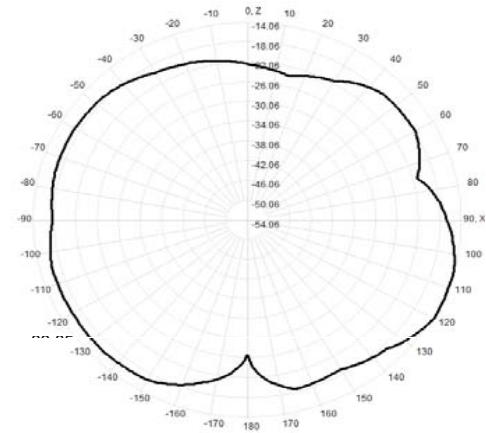
904.0MHz Total(E1-XZ), Max=-14.06dBi
