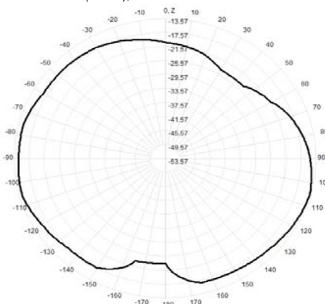
911.0MHz Total(E2-YZ), Max= -14.02dBi
