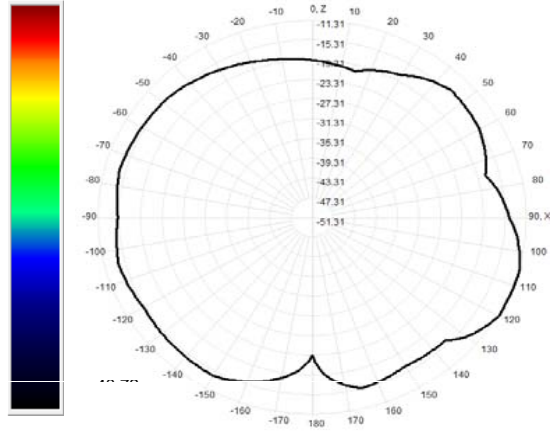
925.0MHz Total(E1-XZ), Max= -11.31dBi
