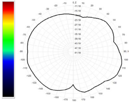
926.0MHz Total(E1-XZ), Max= -11.18dBi
