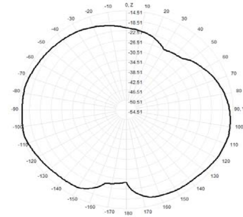
902.0MHz Total(E2-YZ), Max=-15.01dBi
