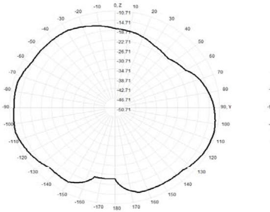
928.0MHz Total(E2-YZ), Max= -11.57dBi
