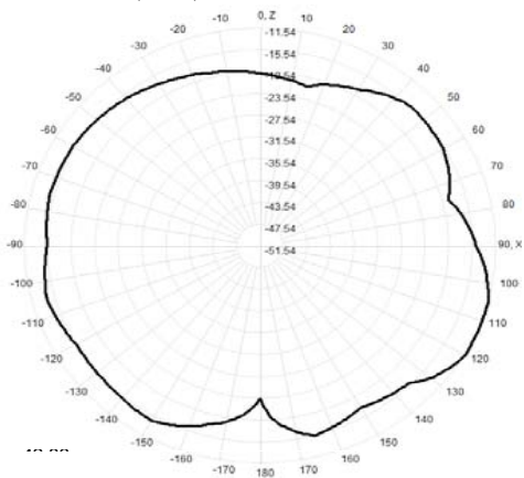
922.0MHz Total(E1-XZ), Max= -11.54dBi
