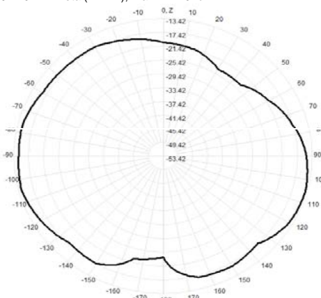
912.0MHz Total(E2-YZ), Max= -14.02dBi
