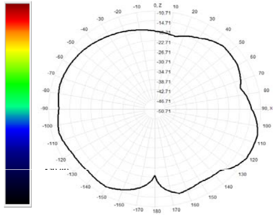
928.0MHz Total(E1-XZ), Max= -10.71dBi
