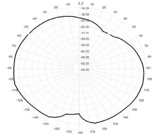
903.0MHz Total(E2-YZ), Max=-14.90dBi
