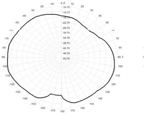
927.0MHz Total(E2-YZ), Max= -11.67dBi
