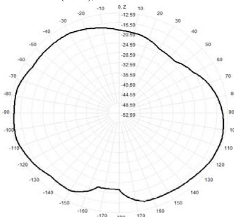
917.0MHz Total(E2-YZ), Max= -13.44dBi
