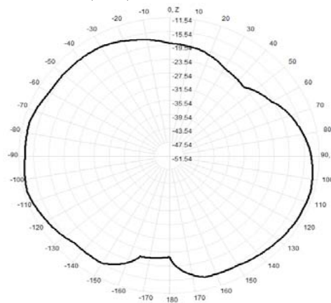
922.0MHz Total(E2-YZ), Max= -12.40dBi
