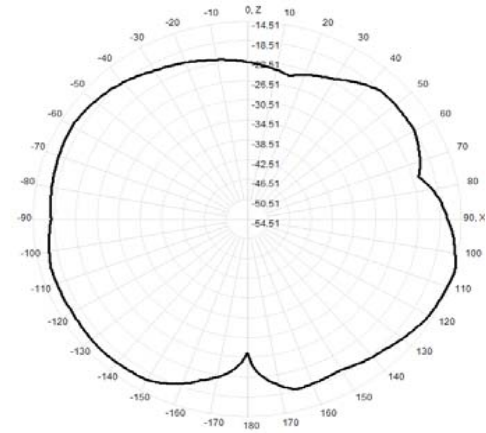
902.0MHz Total(E1-XZ), Max=-14.51dBi
