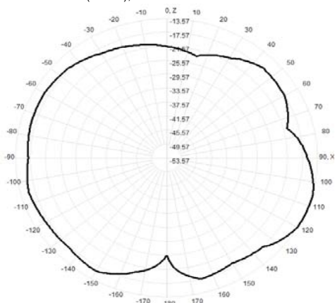
911.0MHz Total(E1-XZ), Max= -13.57dBi
