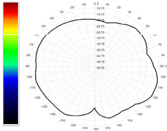
927.0MHz Total(E1-XZ), Max= -10.75dBi
