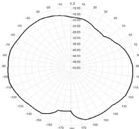
916.0MHz Total(E2-YZ), Max= -13.66dBi
