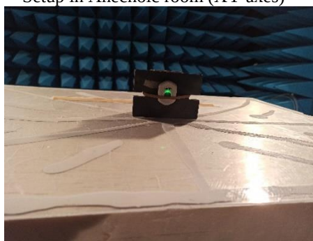
Setup in Anechoic room (Z axes)
