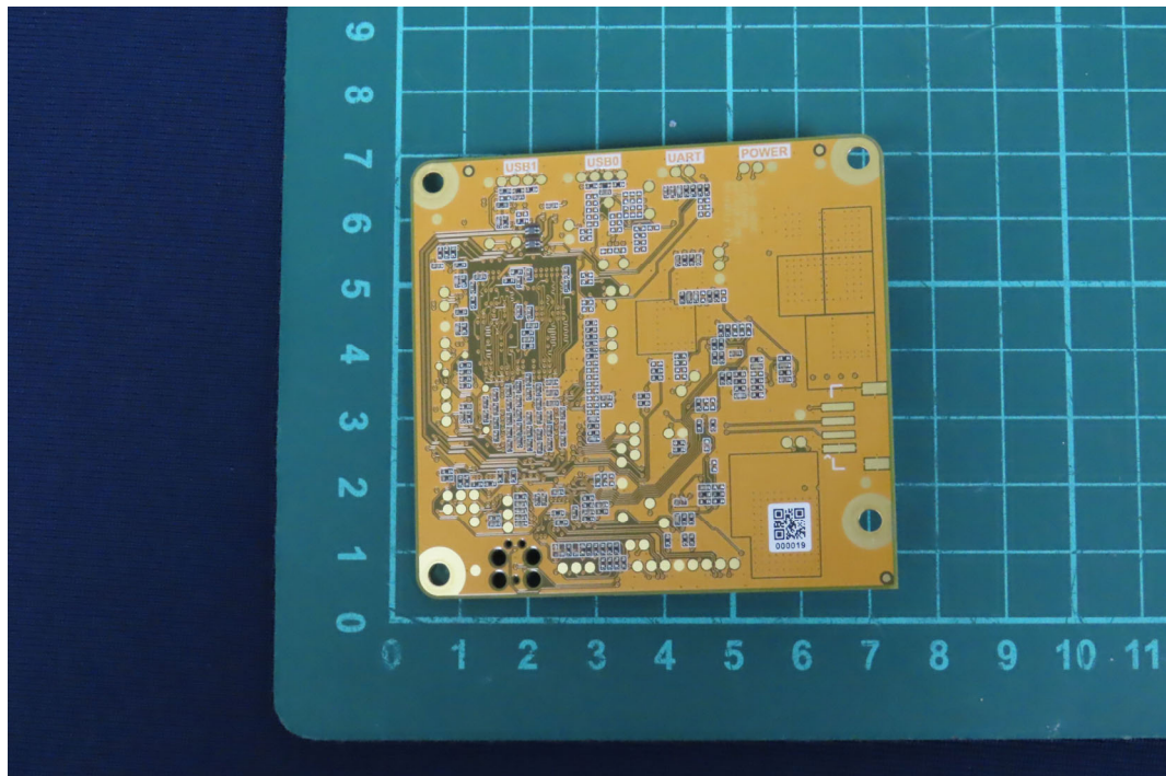
(6) EUT Photo
