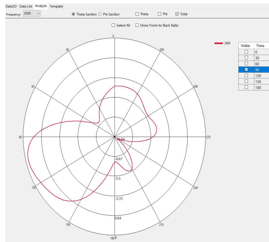
2500MHz
