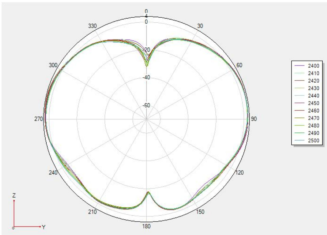
Phi 90 2D 图
