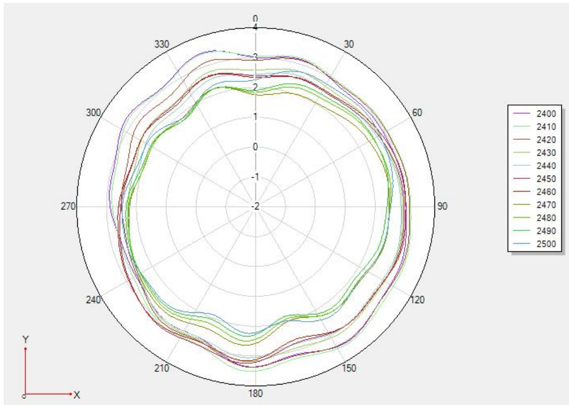
Theta 90 2D 图
