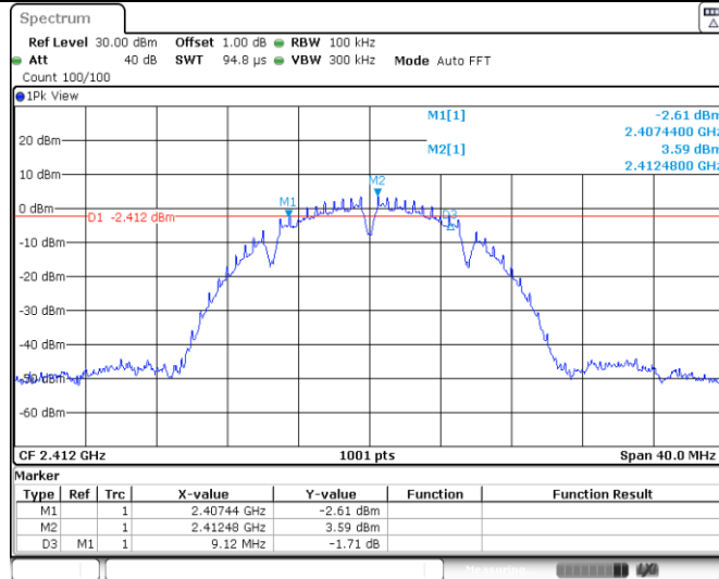
11B_Ant1_2412
