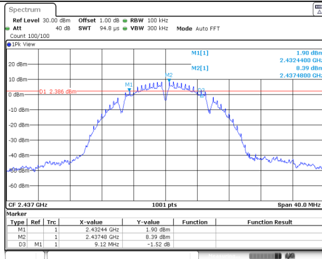
11B_Ant1_2437
