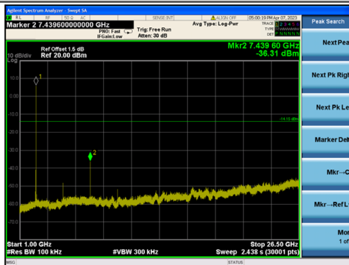
BLE_1Mbps_2480_1000~26500
