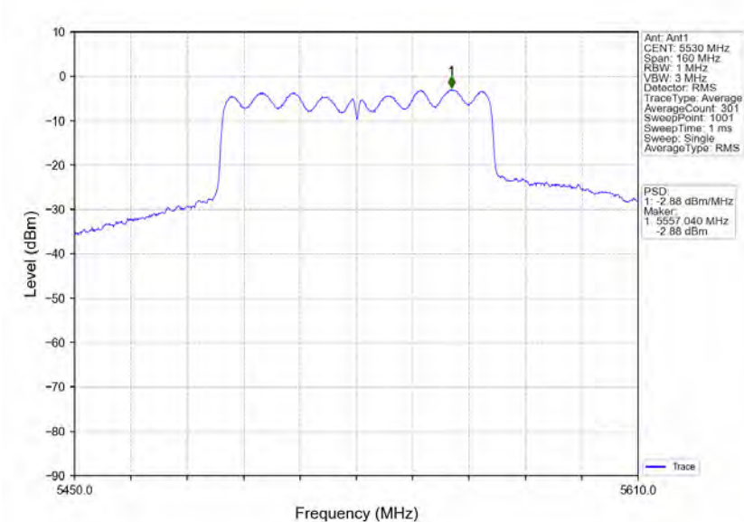
802.11ac(VHT80) LCH_5530MHz_Ant1_NTNV
