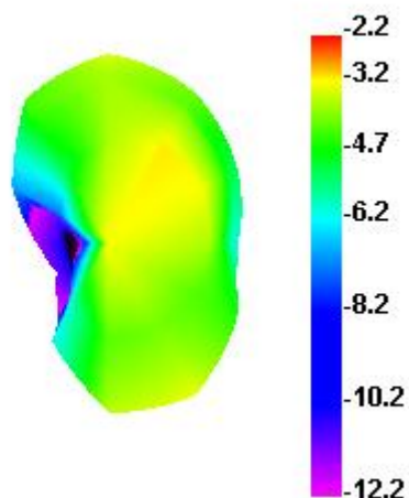
2470.000MHz
