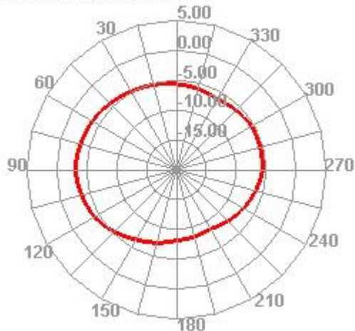
2470.000MHz H
