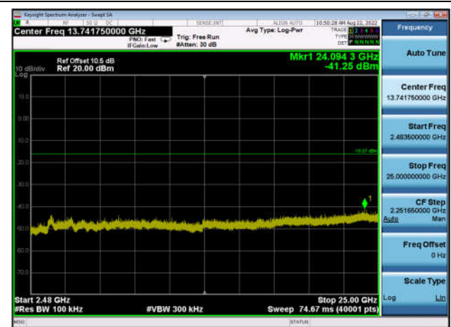
,Plot 4,2483.5MHz~25000MHz-802.11n(HT20),2462MHz,Ant0
