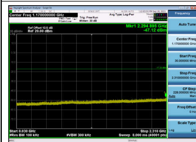
,Plot 3,30MHz~2310MHz-802.11g,2437MHz
