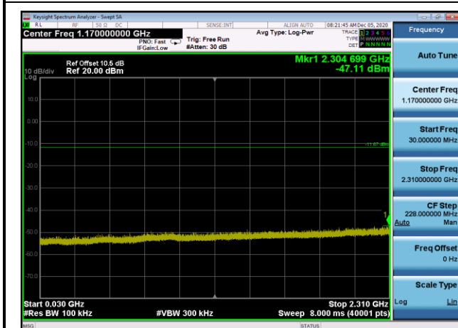
,Plot 3,30MHz~2310MHz-802.11b,2462MHz
