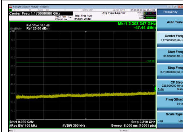
,Plot 3,30MHz~2310MHz-802.11b,2462MHz
