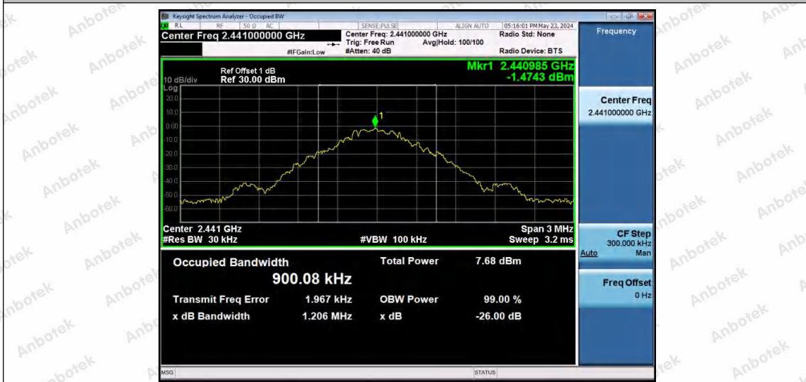
DH5-Ant1-2441
