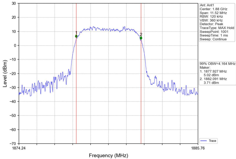
Band2_HSUPA_MCH_1880MHz_Subtest 1_NTNV
