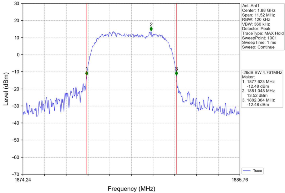
Band2_HSUPA_MCH_1880MHz_Subtest 1_NTNV
