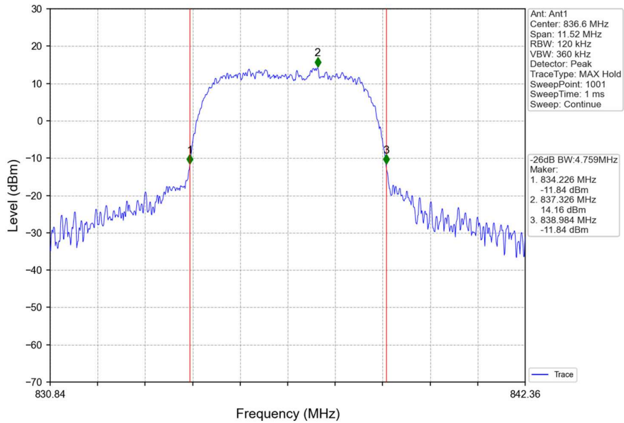
Band5_HSUPA_MCH_836.6MHz_Subtest 1_NTNV
