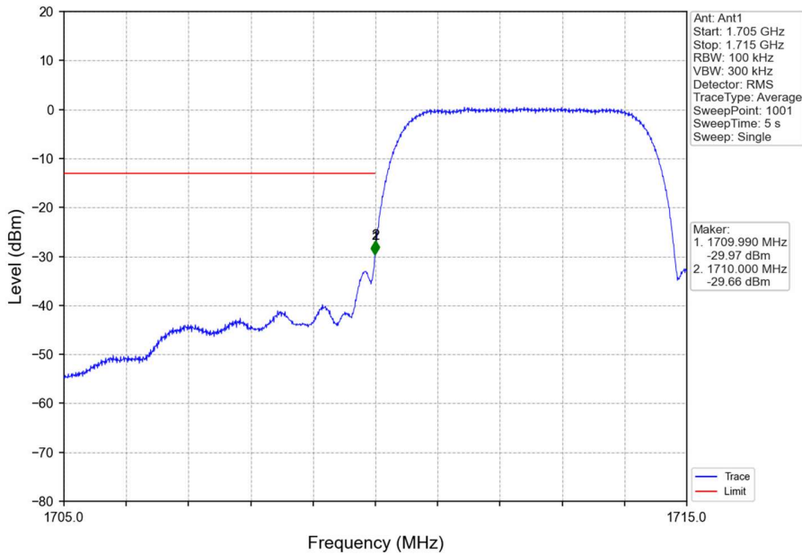
Band4_HSUPA_LCH_1712.4MHz_Subtest 1_NTNV
