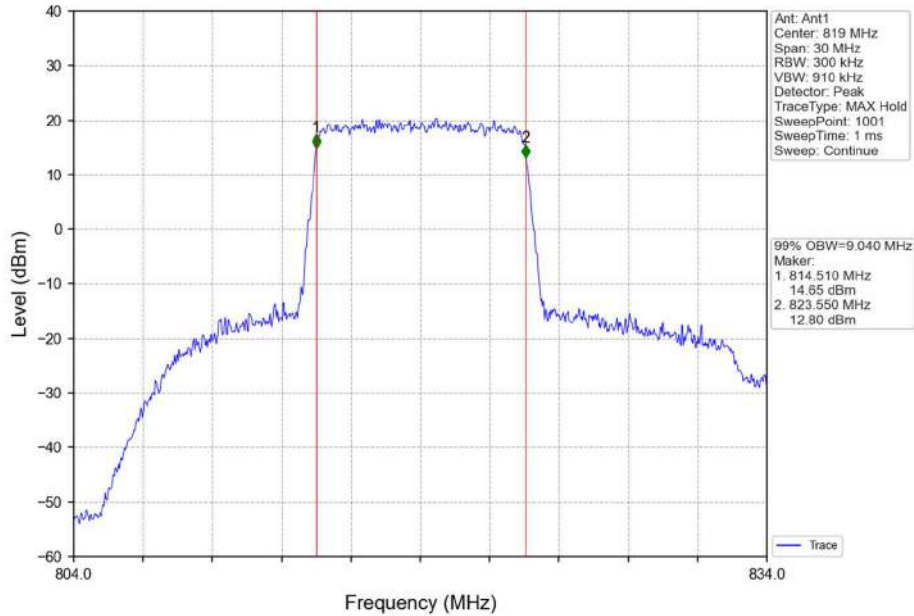
Band26a_10MHz_QPSK_MCH_819MHz_RB_50_0_NTNV
