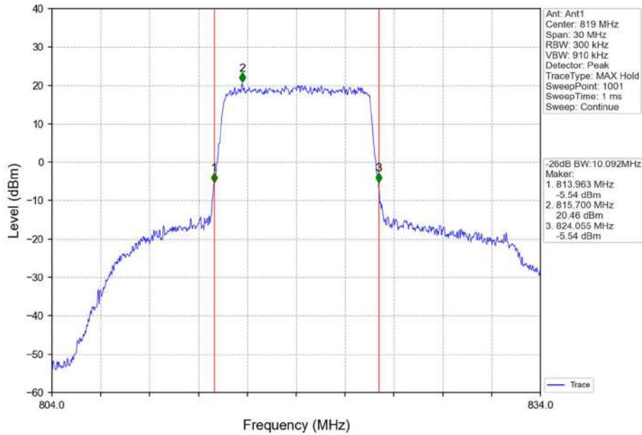
Band26a 10MHz QPSK LCH 819MHz RB 50 0 NTN
