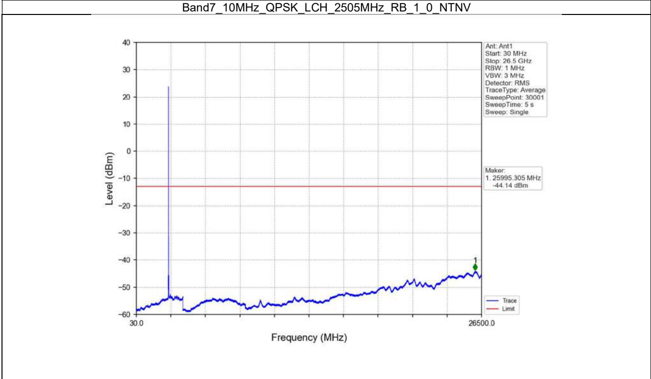
Band7_10MHz_QPSK_LCH_2505MHz_RB_1_0_NTNV
