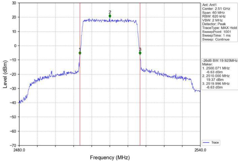
Band7_20MHz_QPSK_LCH_2510MHz_RB_100_0_NTNV
