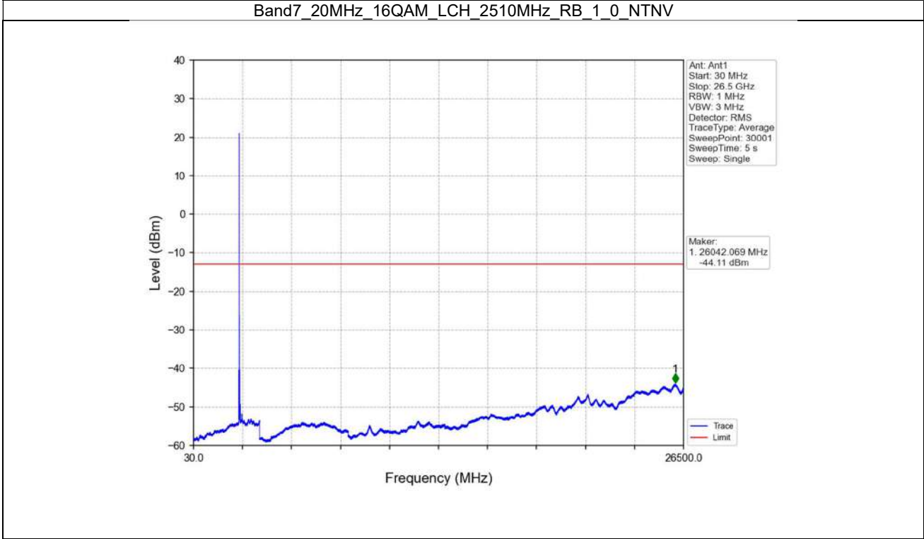
Band7_20MHz_16QAM_LCH_2510MHz_RB_1_0_NTNV
