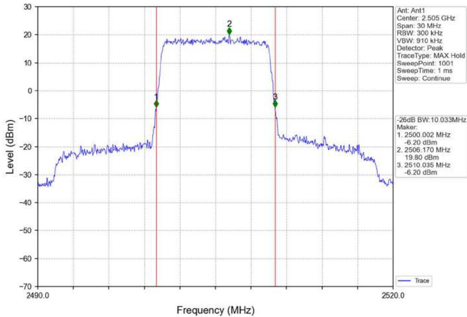
Band7_10MHz_QPSK_LCH_2505MHz_RB_50_0_NTNV
