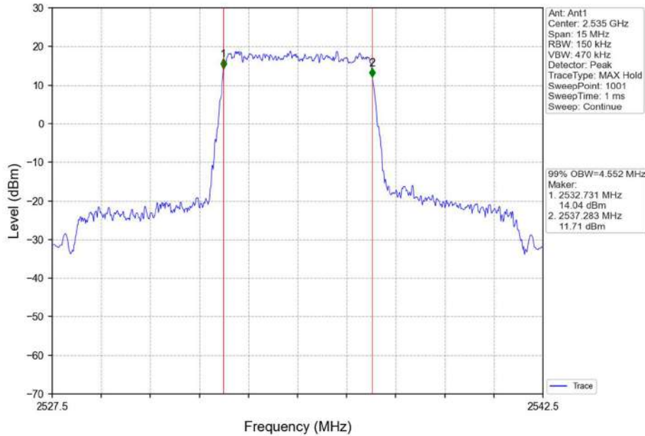
Band7_5MHz_QPSK_MCH_2535MHz_RB_25_0_NTNV
