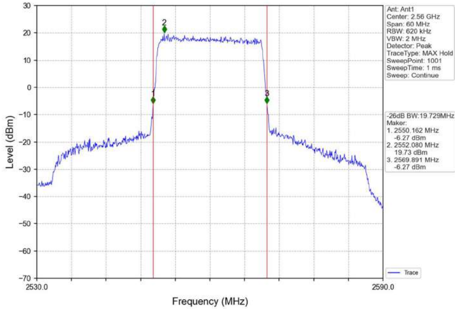
Band7_20MHz_QPSK_HCH_2560MHz_RB_100_0_NTNV
