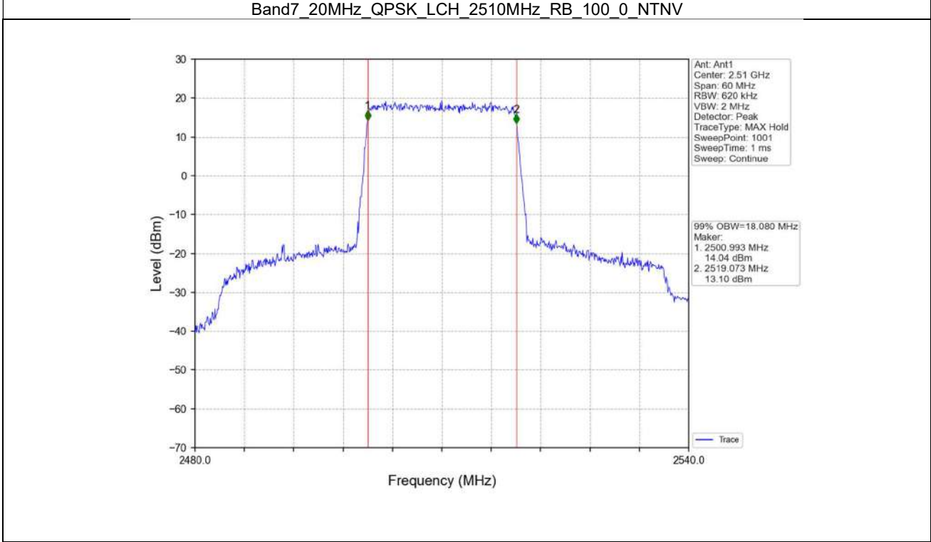
Band7_20MHz_QPSK_LCH_2510MHz_RB_100_0_NTNV
