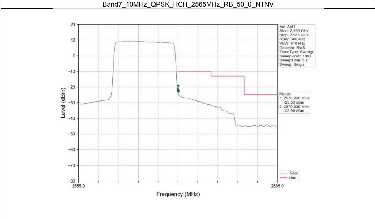
Band7_10MHz_QPSK_HCH_2565MHz_RB_50_0_NTNV
