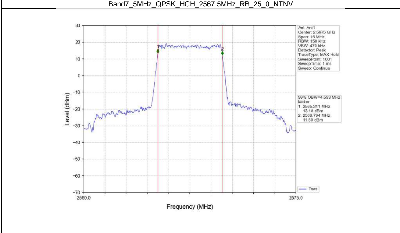
Band7_5MHz_QPSK_HCH_2567.5MHz_RB_25_0_NTNV
