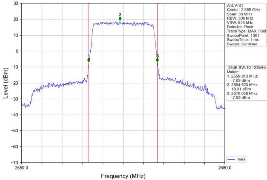
Band7_10MHz_QPSK_HCH_2565MHz_RB_50_0_NTNV
