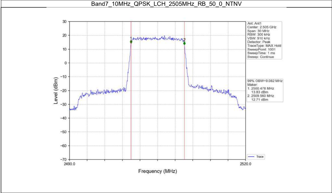
Band7_10MHz_QPSK_LCH_2505MHz_RB_50_0_NTNV
