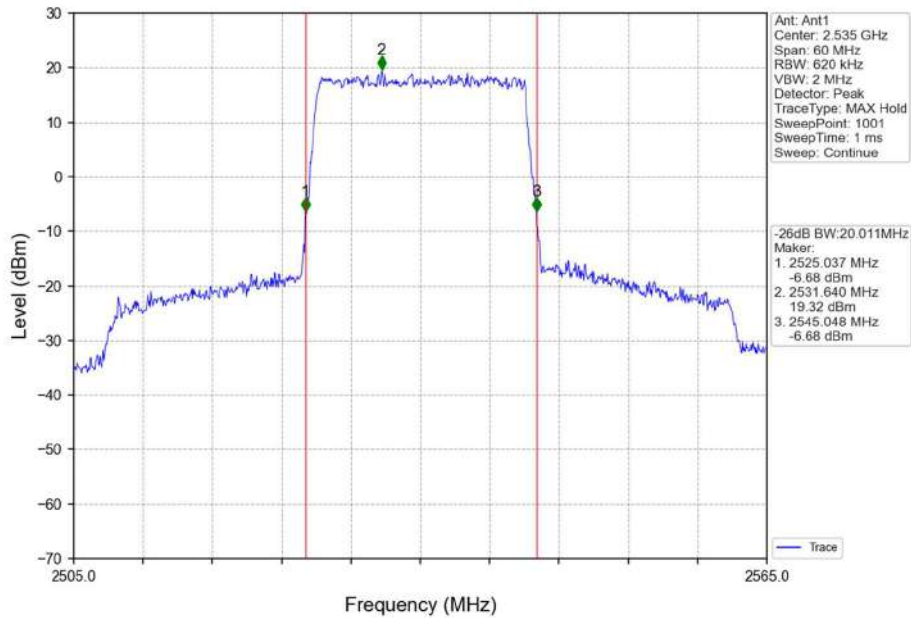
Band7_20MHz_QPSK_MCH_2535MHz_RB_100_0_NTNV
