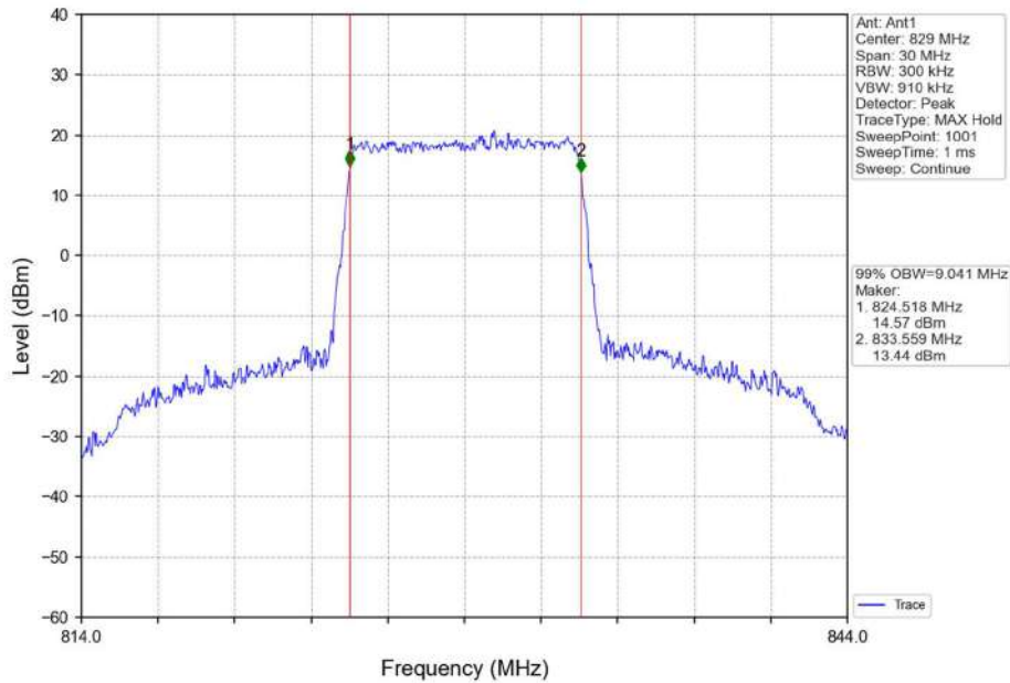
Band5_10MHz_QPSK_LCH_829MHz_RB_50_0_NTNV
