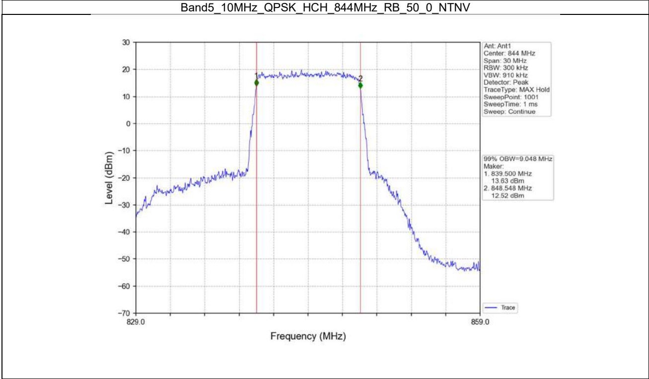
Band5_10MHz_QPSK_HCH_844MHz_RB_50_0_NTNV
