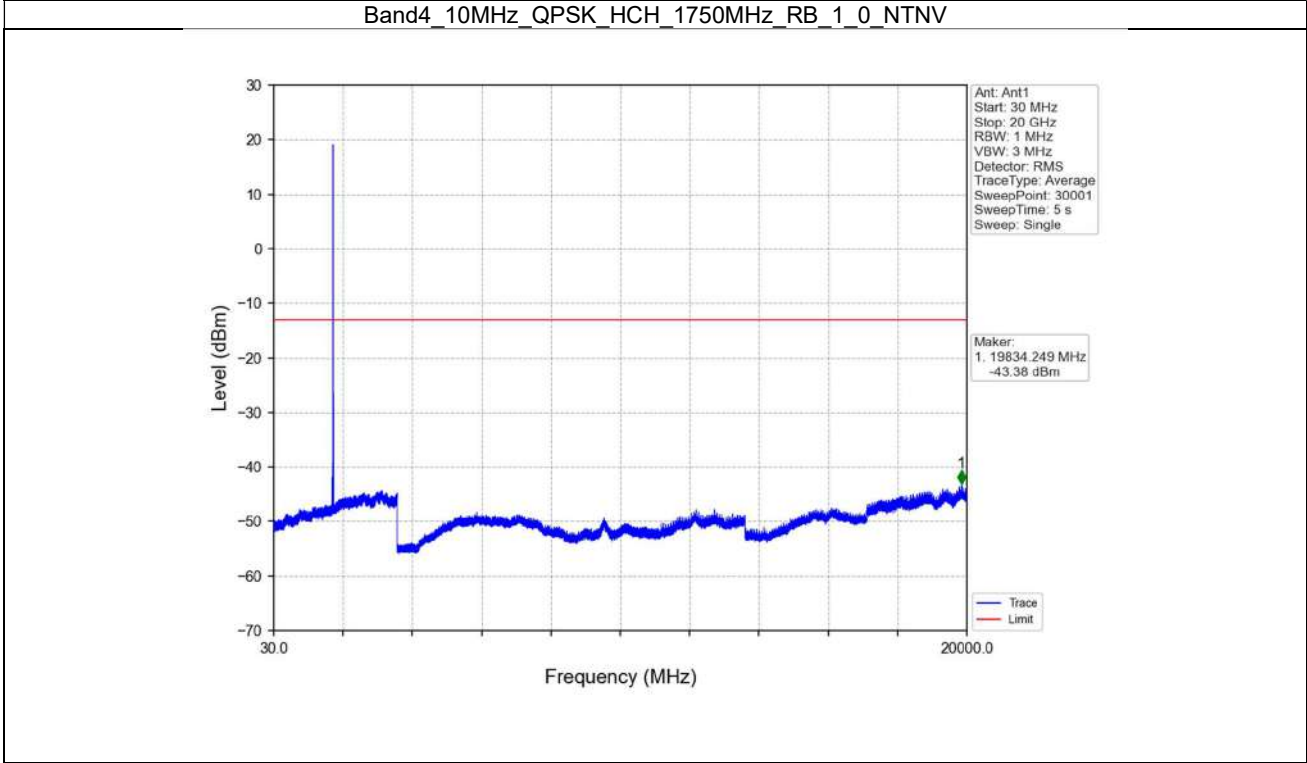
Band4_10MHz_QPSK_HCH_1750MHz_RB_1_0_NTNV
