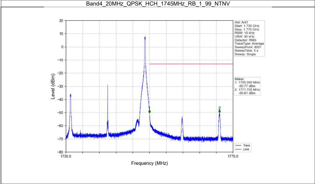
Band4_20MHz_QPSK_HCH_1745MHz_RB_1_99_NTNV
