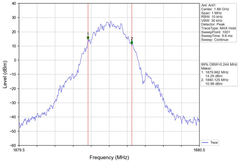
PCS1900_GSM_MCH_1880MHz_GSM_NTNV
