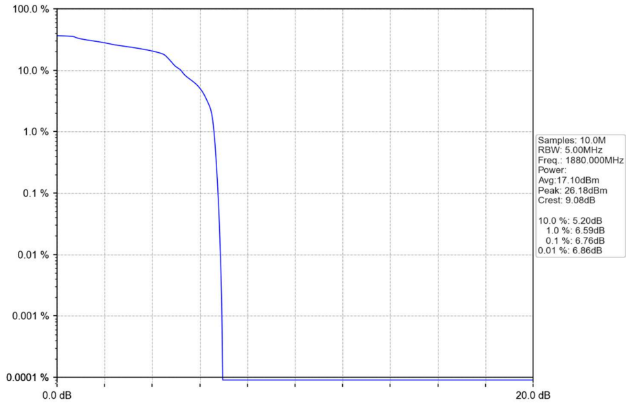
PCS1900_EGPRS_MCH_1880MHz_4_TX Slots_NTNV
