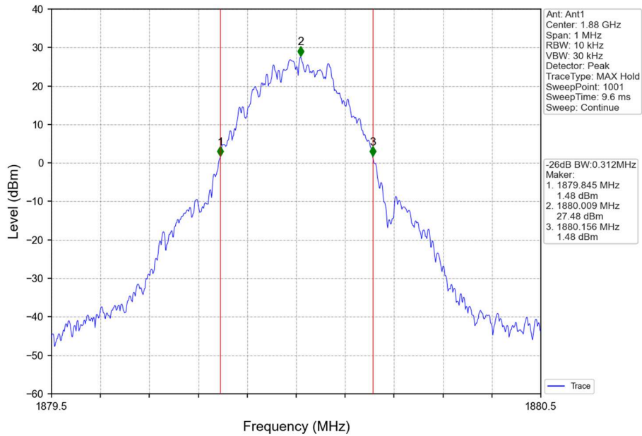
PCS1900_GSM_MCH_1880MHz_GSM_NTNV
