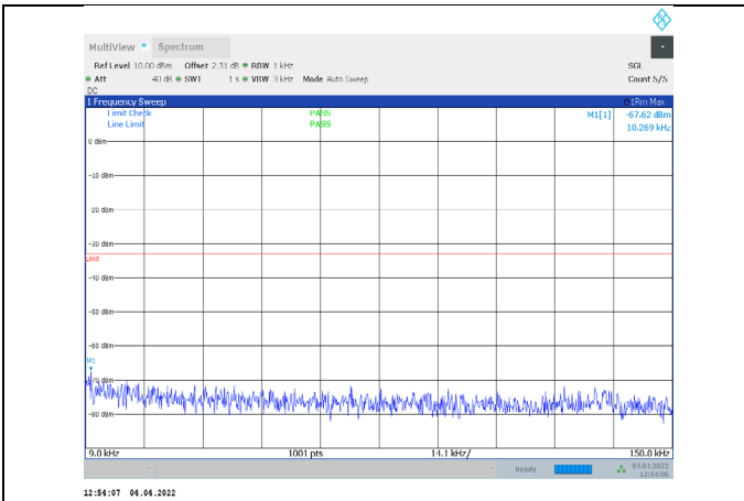
1-N71-PC3-15-20-L-1-CP-QPSK-Edge_1RB_Left-1@0 -0.009-0.15-Ant1--67.62--33-PASS
