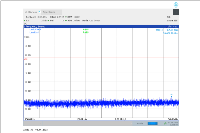
1-N71-PC3-15-15-H-2-CP-QPSK-Edge_1RB_Right-1@ 78-0.15-30-Ant1--67.16--23-PASS
