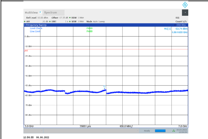
1-N71-PC3-15-20-L-1-CP-QPSK-Edge_1RB_Left-1@0 -3000-7000-Ant1--53.74--13-PASS
