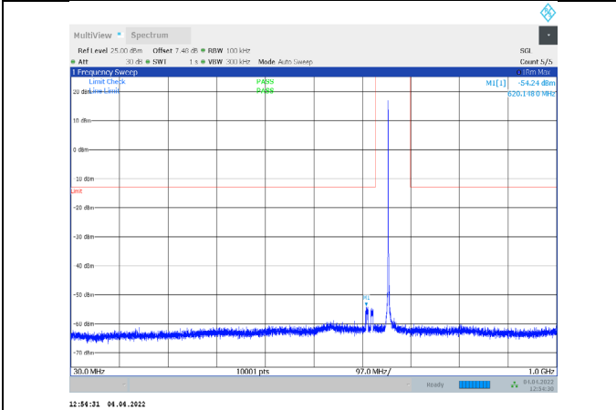
1-N71-PC3-15-20-L-1-CP-QPSK-Edge_1RB_Left-1@0 -30-1000-Ant1--54.24--13-PASS
