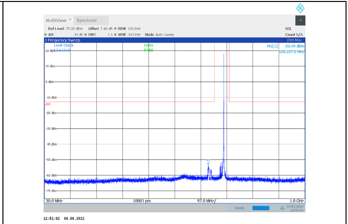
1-N71-PC3-15-15-H-2-CP-QPSK-Edge_1RB_Right-1@ 78-30-1000-Ant1--53.49--13-PASS
