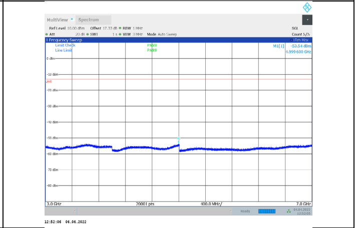
1-N71-PC3-15-15-H-2-CP-QPSK-Edge_1RB_Right-1@ 78-3000-7000-Ant1--53.54--13-PASS
