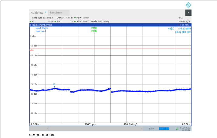
1-N71-PC3-15-20-M-2-CP-QPSK-Edge_1RB_Right-1@10 5-3000-7000-Ant1--53.22--13-PASS
