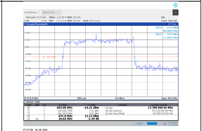
1-N71-PC3-15-20-L-6-DFT-QPSK-Outer_Full-100@0-Ant1-17.701-18.640-≤20-PASS
