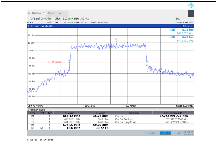
1-N71-PC3-15-20-L-1-CP-QPSK-Outer_Full-100@0-Ant 1-17.756-18.600-≤20-PASS
