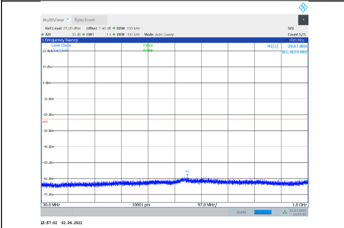
1-N66-PC3-15-15-M-1-CP-QPSK-Edge_1RB_Left-1@0 -30-1000-Ant1--58.67--23-PASS
