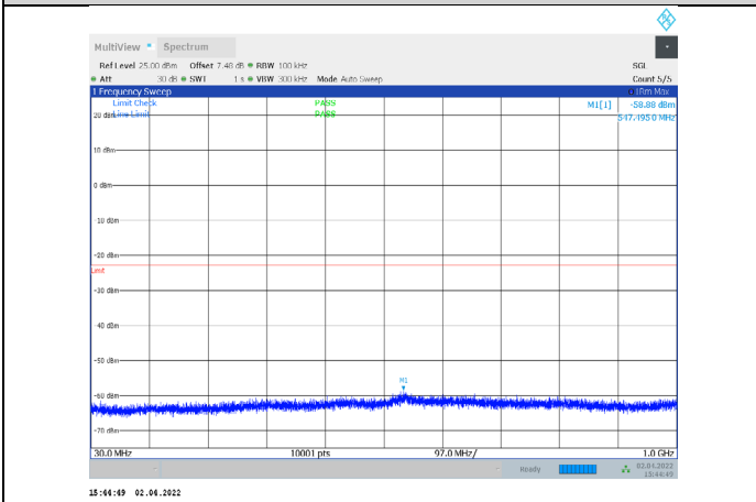
1-N66-PC3-15-5-M-2-CP-QPSK-Edge_1RB_Right-1@2 4-30-1000-Ant1--58.88--23-PASS
