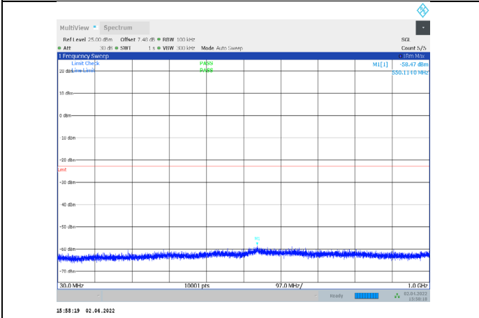
1-N66-PC3-15-15-M-2-CP-QPSK-Edge_1RB_Right-1@ 78-30-1000-Ant1--58.47--23-PASS
