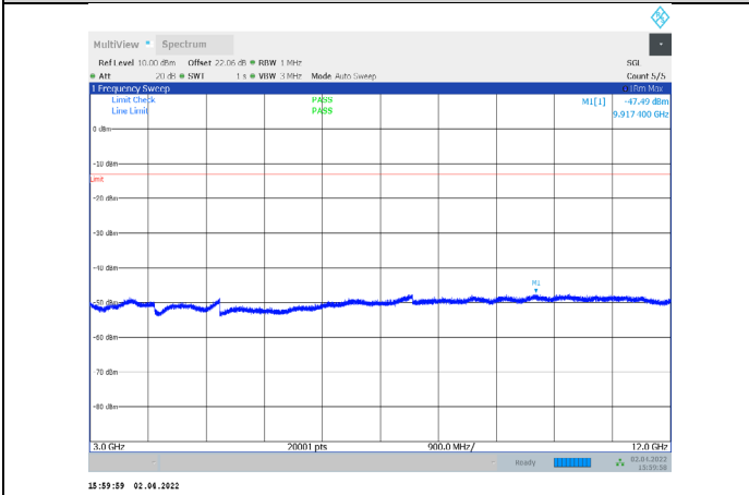
1-N66-PC3-15-15-M-3-CP-QPSK-Outer_Full-79@0-30 00-12000-Ant1--47.49--13-PASS
