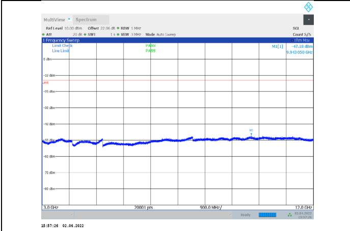
1-N66-PC3-15-15-M-1-CP-QPSK-Edge_1RB_Left-1@0 -3000-12000-Ant1--47.18--13-PASS
