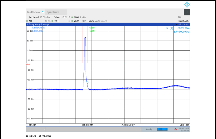
1-N66-PC3-15-15-L-3-CP-QPSK-Outer_Full-79@0-1000- 3000-Ant1--35.26--13-PASS
