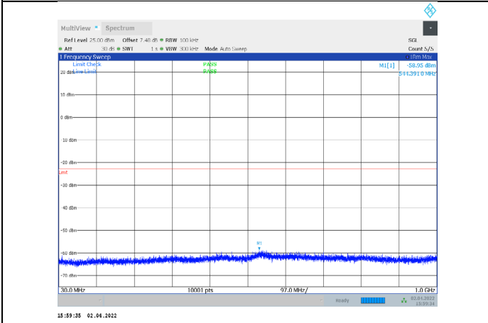
1-N66-PC3-15-15-M-3-CP-QPSK-Outer_Full-79@0-30- 1000-Ant1--58.95--23-PASS
