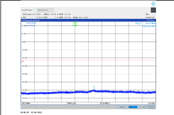
1-N66-PC3-15-5-H-2-CP-QPSK-Edge_1RB_Right-1@2 4-30-1000-Ant1--58.78--23-PASS
