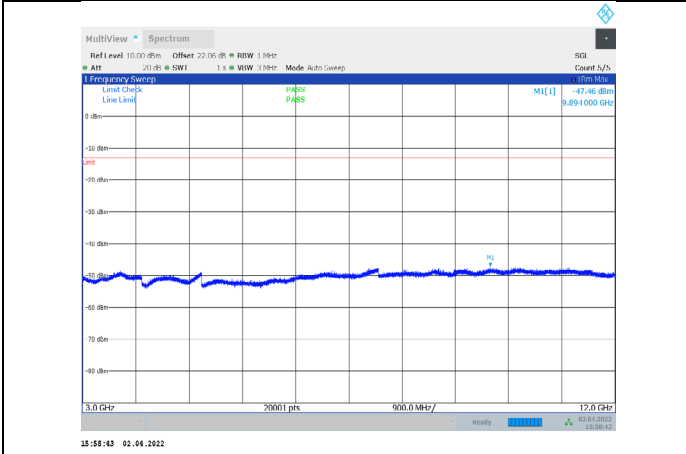
1-N66-PC3-15-15-M-2-CP-QPSK-Edge_1RB_Right-1@ 78-3000-12000-Ant1--47.46--13-PASS
