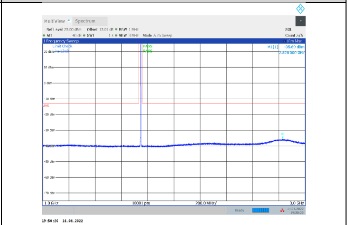
1-N66-PC3-15-5-M-2-CP-QPSK-Edge_1RB_Right-1@2 4-1000-3000-Ant1--35.69--13-PASS
