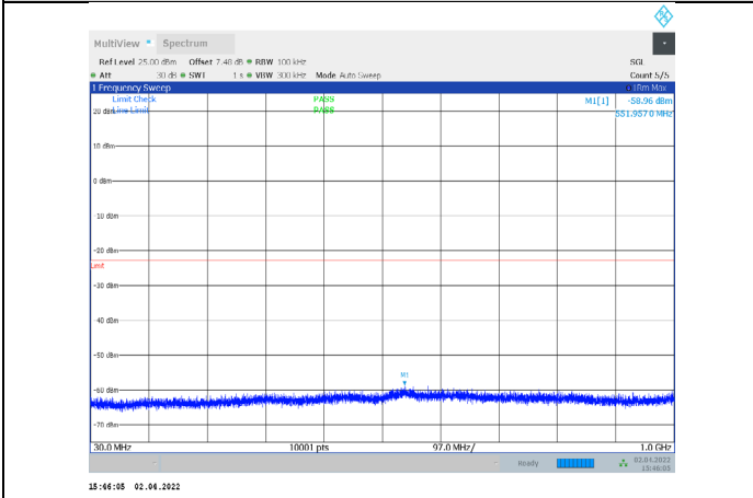
1-N66-PC3-15-5-M-3-CP-QPSK-Outer_Full-25@0-30-1 000-Ant1--58.96--23-PASS
