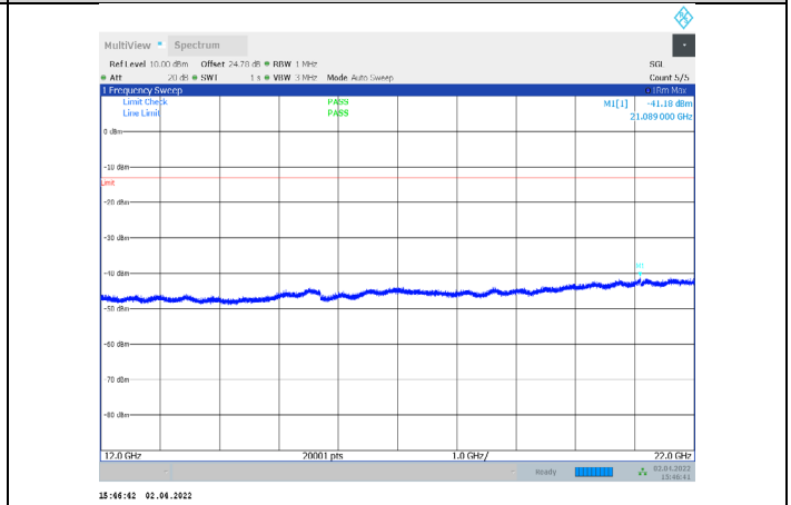
1-N66-PC3-15-5-M-3-CP-QPSK-Outer_Full-25@0-1200 0-22000-Ant1--41.18--13-PASS
