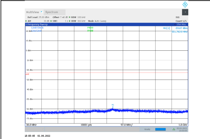
1-N66-PC3-15-15-L-3-CP-QPSK-Outer_Full-79@0-30- 1000-Ant1--59.07--23-PASS
