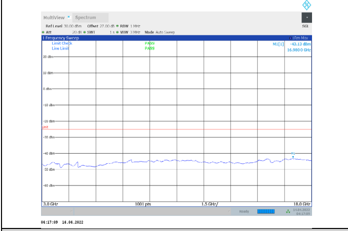
1-N41-PC3-30-100-L-2-CP-QPSK-Edge_1RB_Right-1 @272-3000-18000-Ant1--43.13--25-PASS
