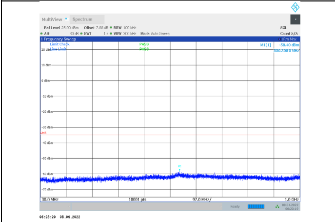
1-N7-PC3-15-15-L-3-CP-QPSK-Outer_Full-79@0-30-1 000-Ant1--58.40--35-PASS
