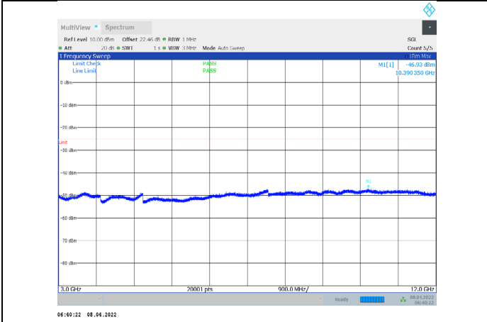
1-N7-PC3-15-20-M-2-CP-QPSK-Edge_1RB_Right-1@1 05-3000-12000-Ant1--46.93--25-PASS
