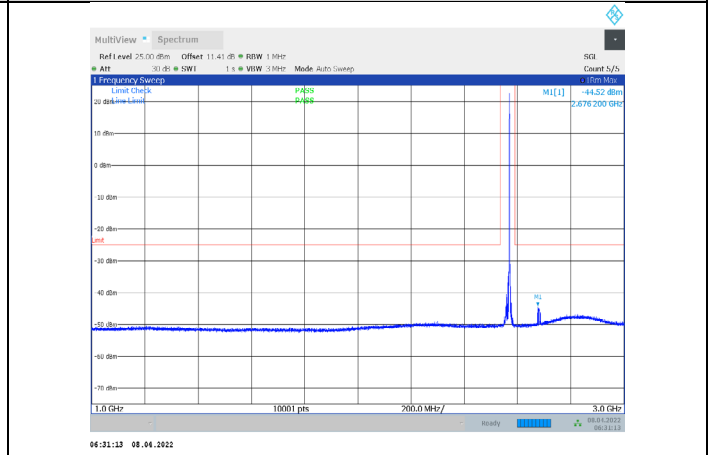
1-N7-PC3-15-15-H-2-CP-QPSK-Edge_1RB_Right-1@7 8-1000-3000-Ant1--44.52--25-PASS
