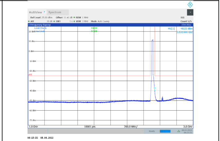
1-N7-PC3-15-15-L-3-CP-QPSK-Outer_Full-79@0-1000-3 000-Ant1--40.53--25-PASS
